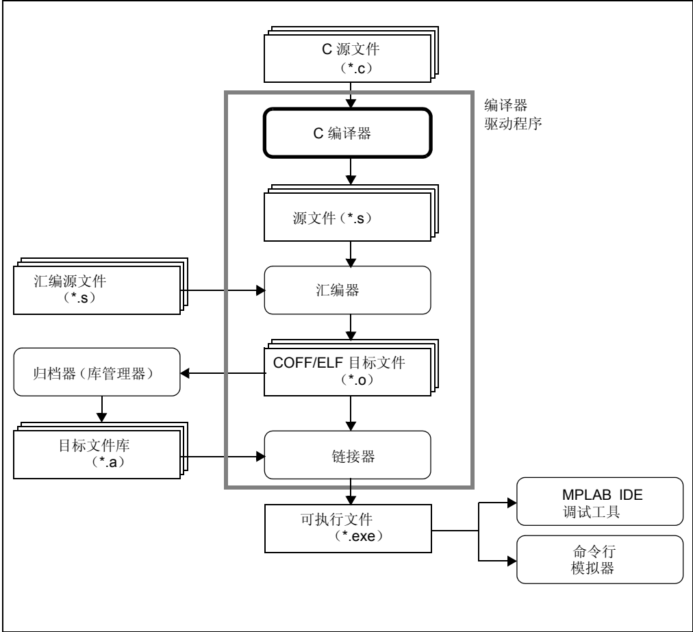
图 1-1: 软件开发工具数据流图
