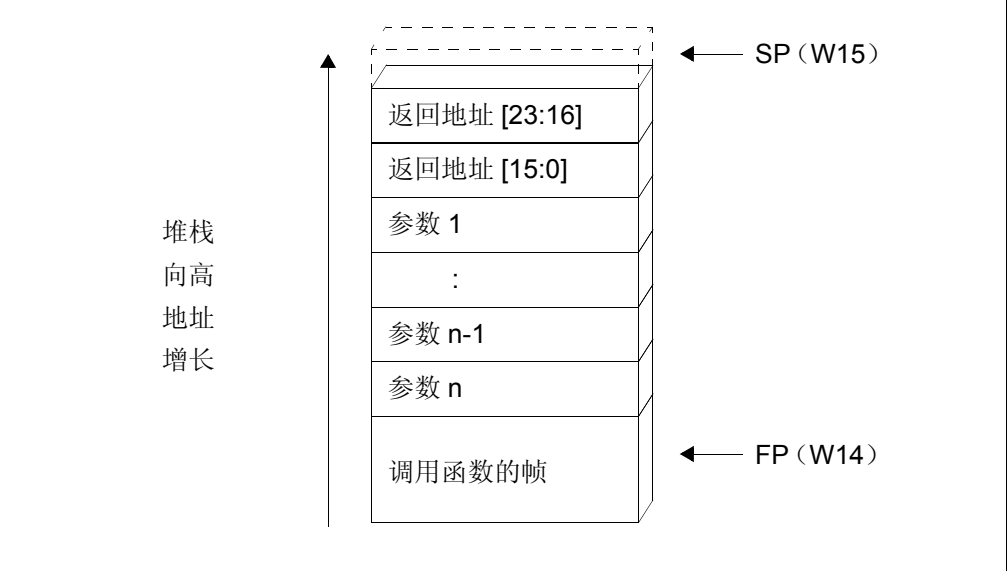
图 4-4: CALL 或 RCALL
