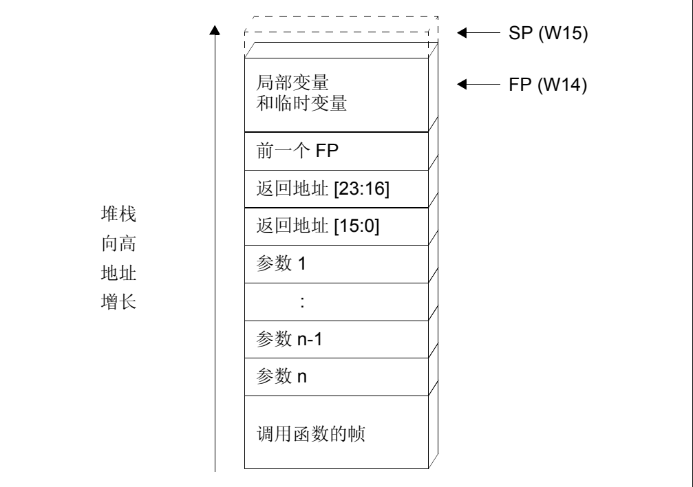
图 4-5: 被调用函数的空间分配
