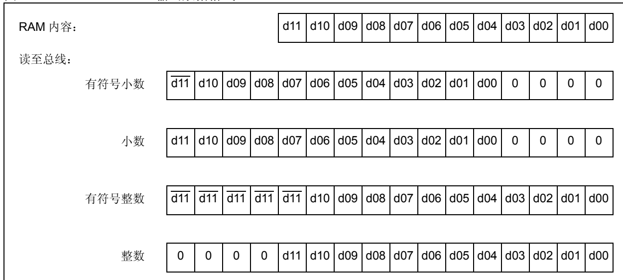
图 19-5: ADC 输出数据格式
