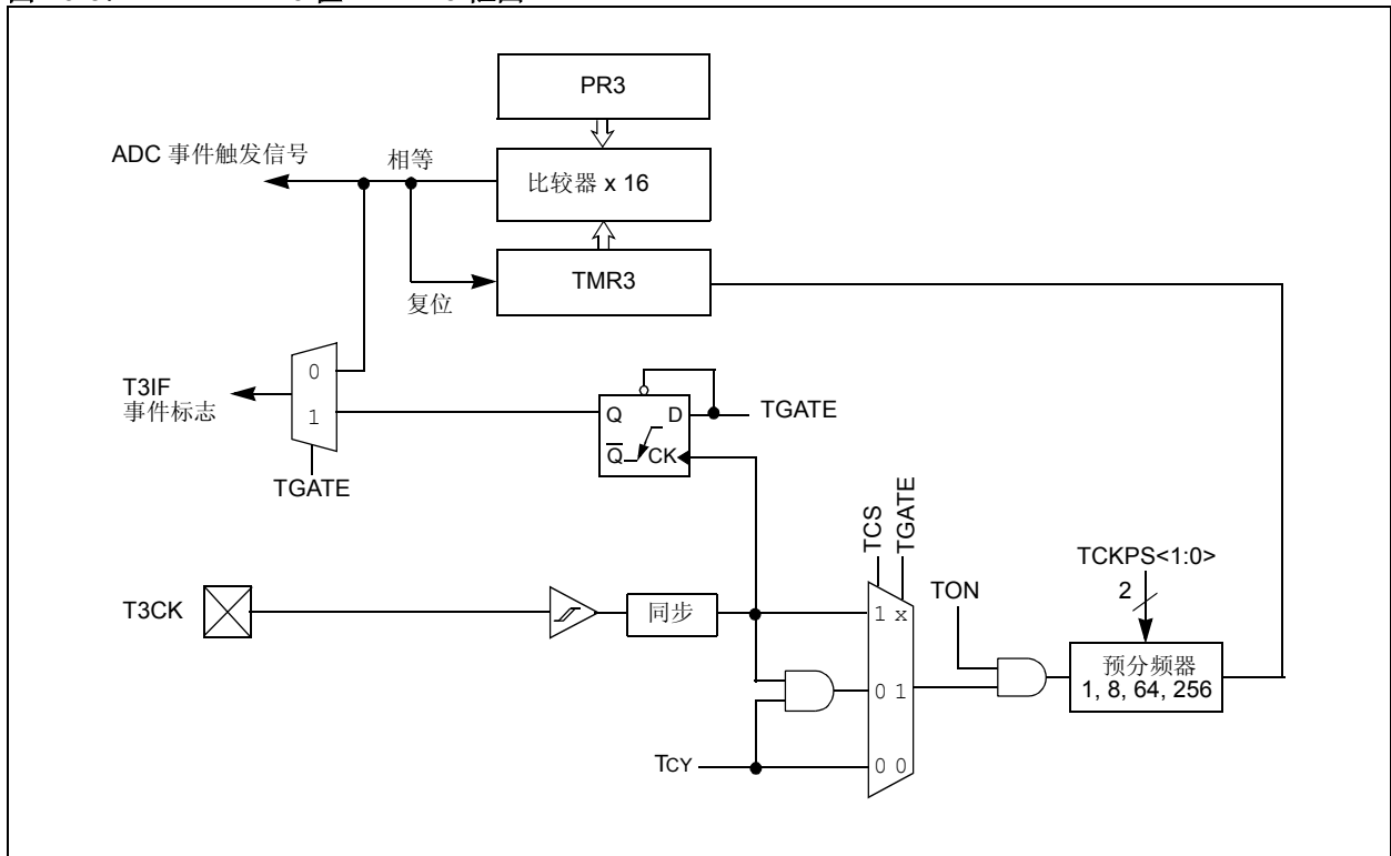
图 10-3: 16 位 TIMER3 框图
