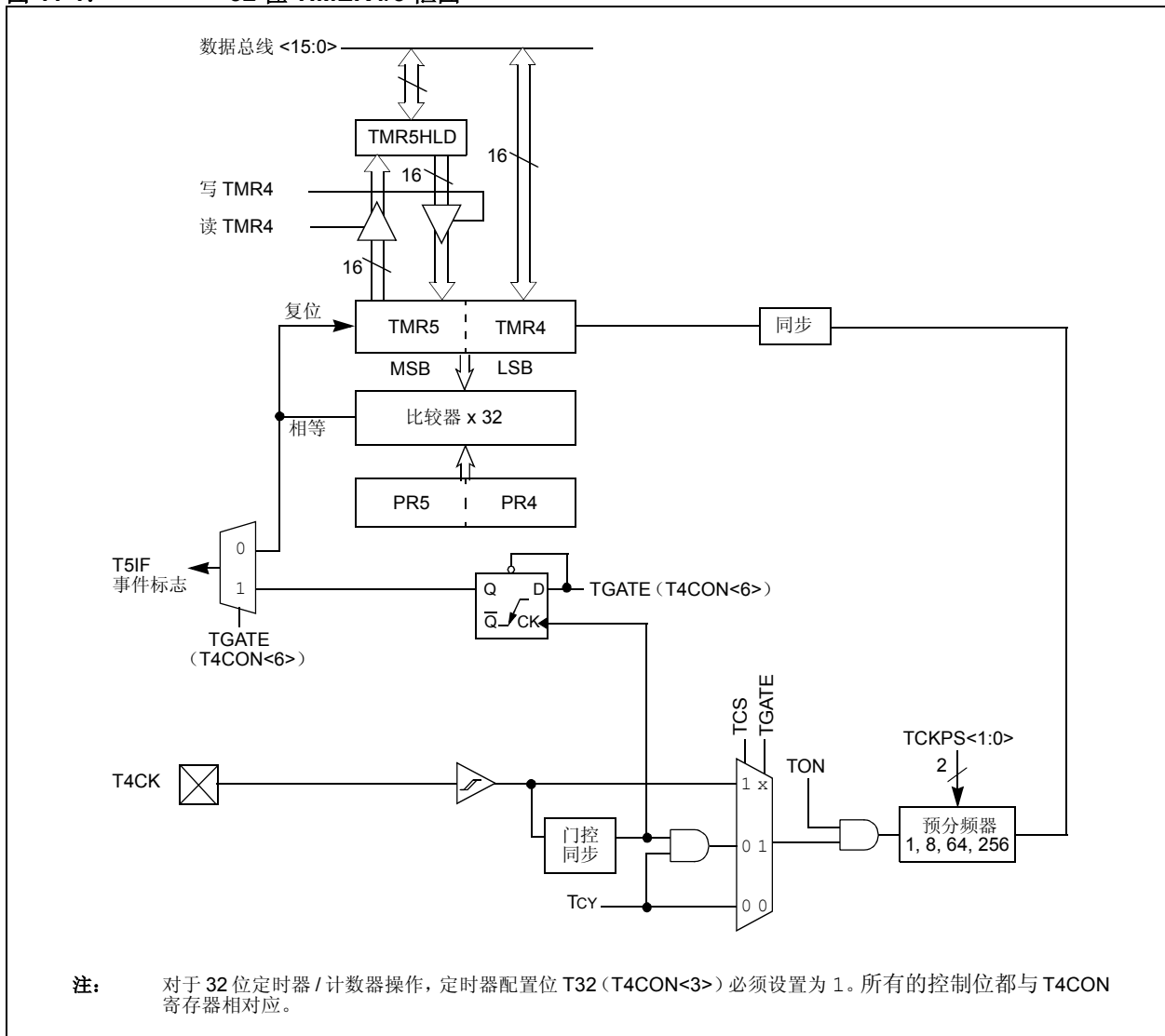
图 11-1: 32 位 TIMER4/5 框图
