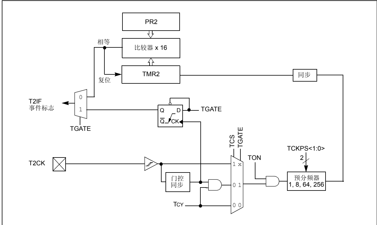
图 10-2: 16 位 TIMER2 框图
