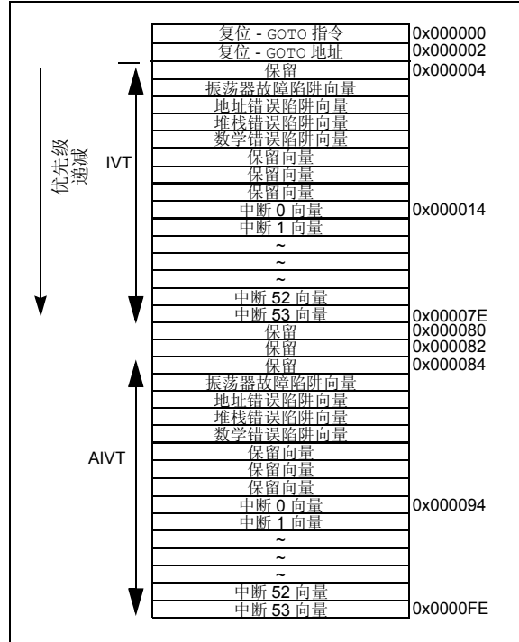
图 5-1: 陷阱向量
