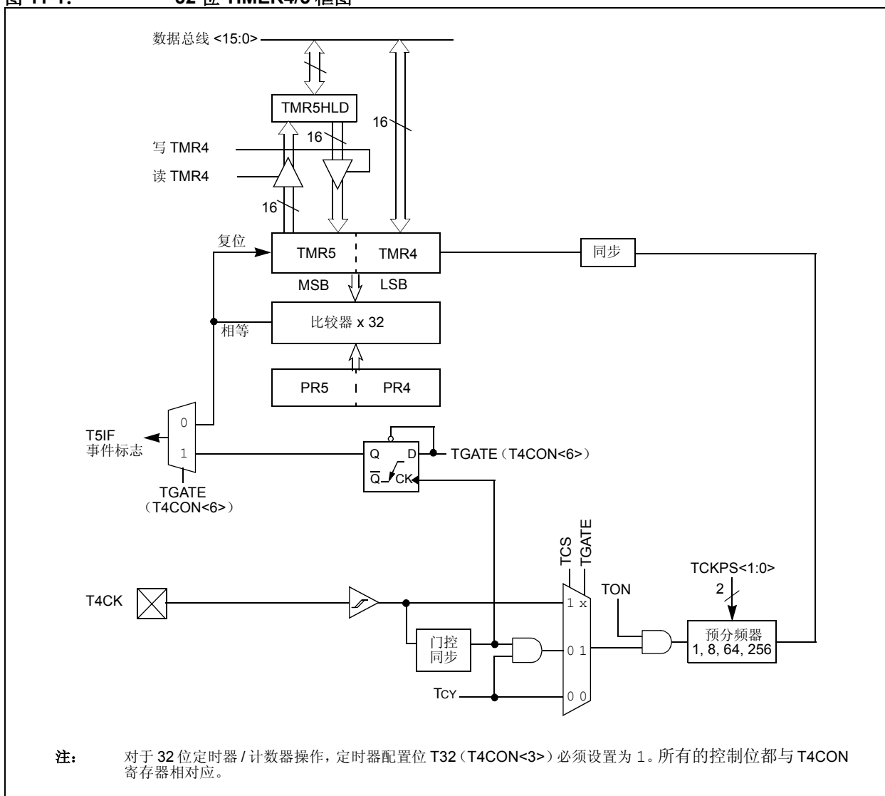
图 11-1: 32 位 TIMER4/5 框图
