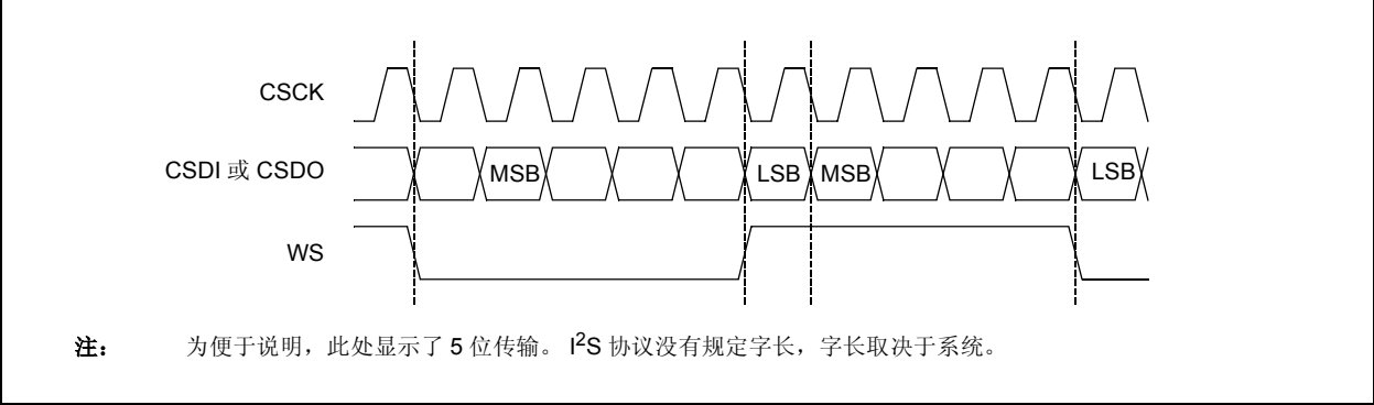
图 18-4: I 2 S 接口帧 同步时序
