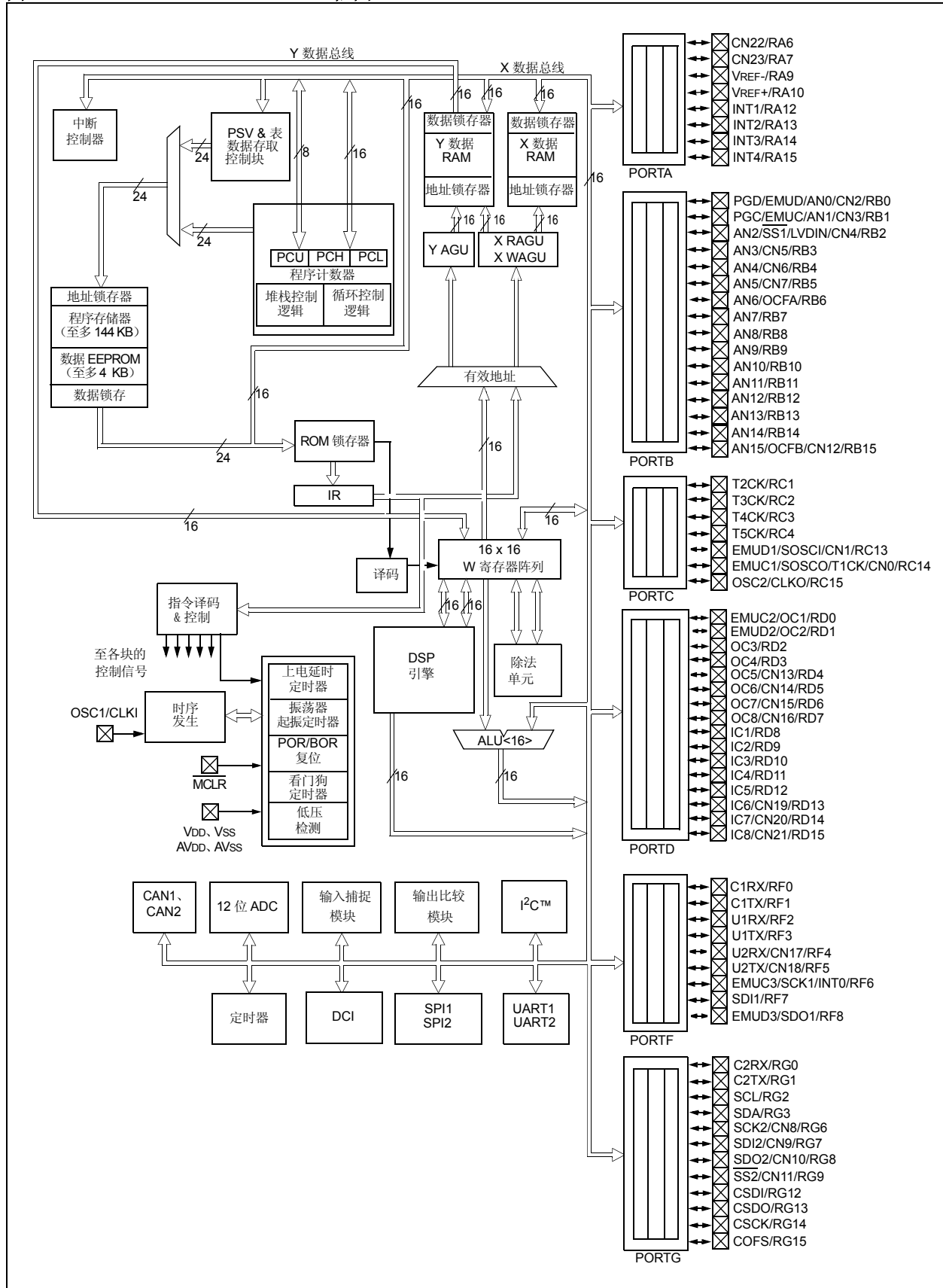
图 1-2: dsPIC30F6013A/6014A 框图
