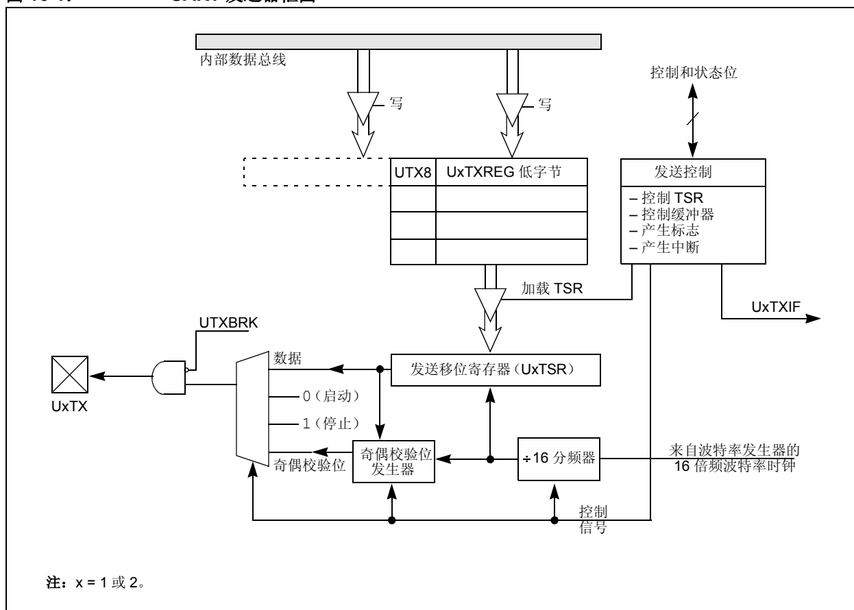
图 16-1: UART 发送器框图
