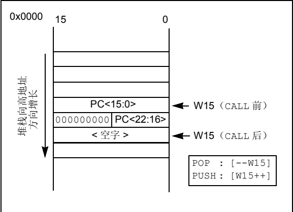
图 3-11： CALL 堆栈帧
