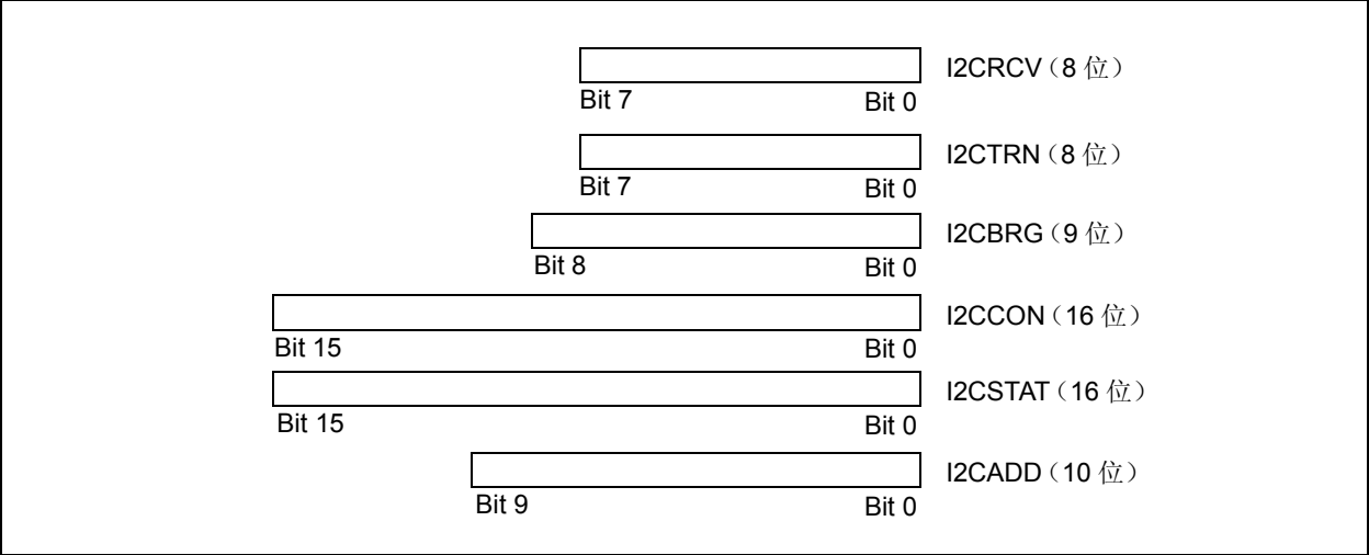
图 15-1: 编程模型
