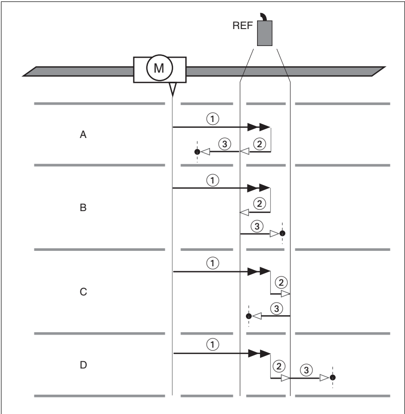
图 8.12 沿正方向朝向基准开关的基准点定位运行
