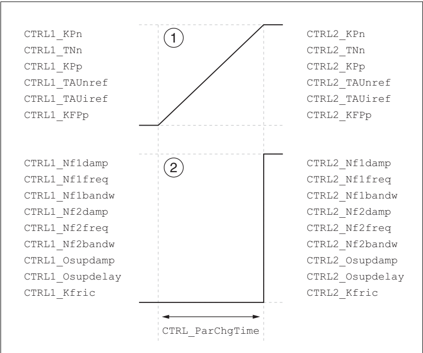
图 8.25 切换控制器参数数组的时序图
