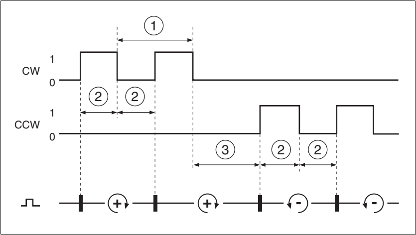
图 3.9 时间图和 “CW/CCW”
