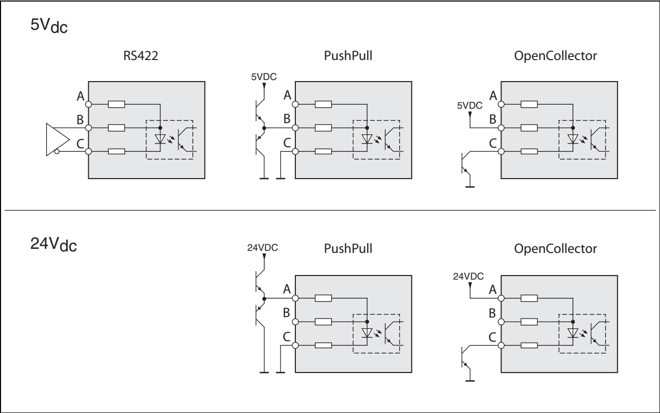
图 3.6 信号输入线路图：RS422、推挽式和集电极开路
