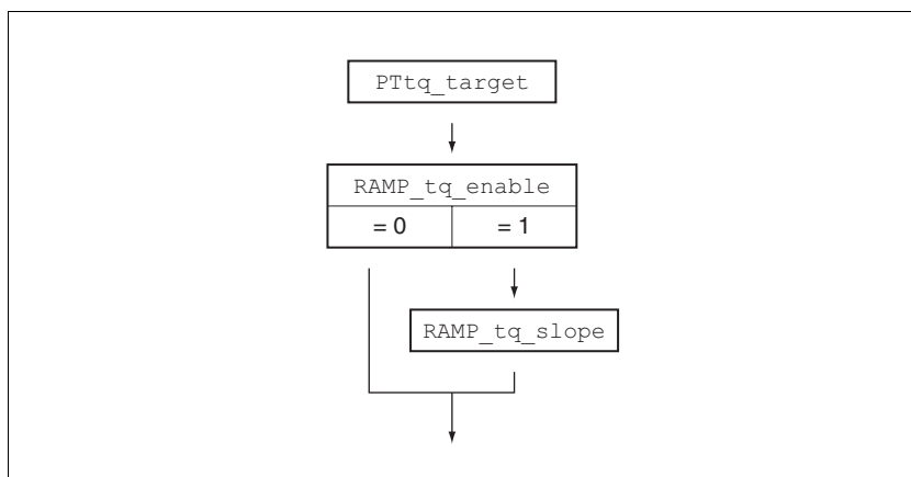
图 8.7 可设置参数的概况
