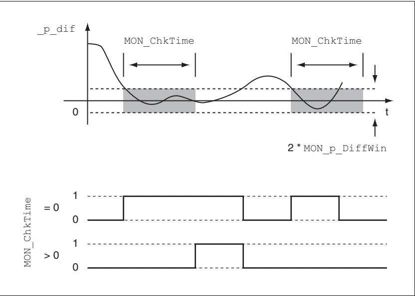
图 8.35 位置偏差窗口
