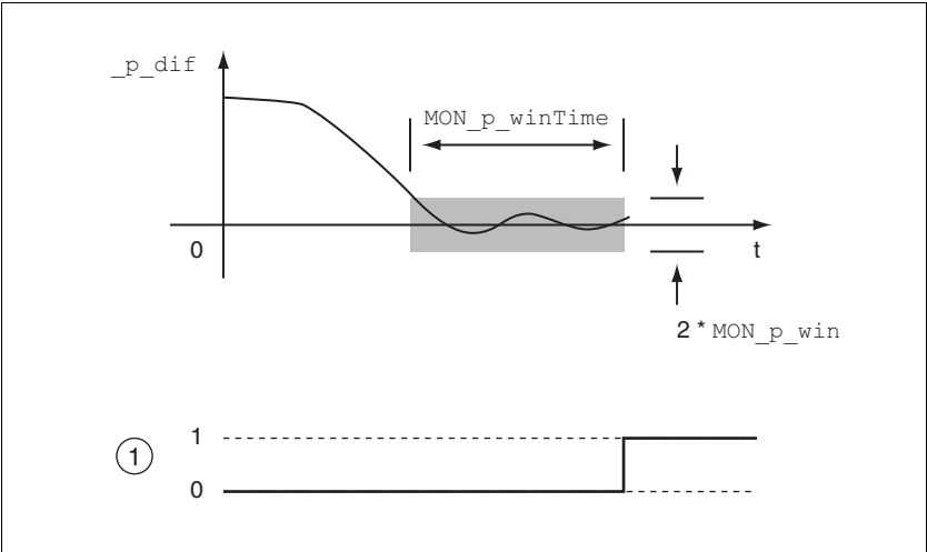
图 8.33 停止范围
