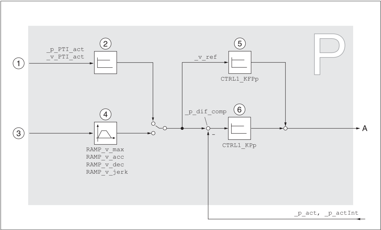
图 8.21 位置控制器
