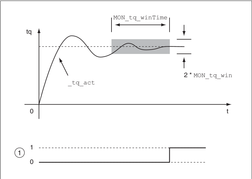
图 8.31 转矩窗口
