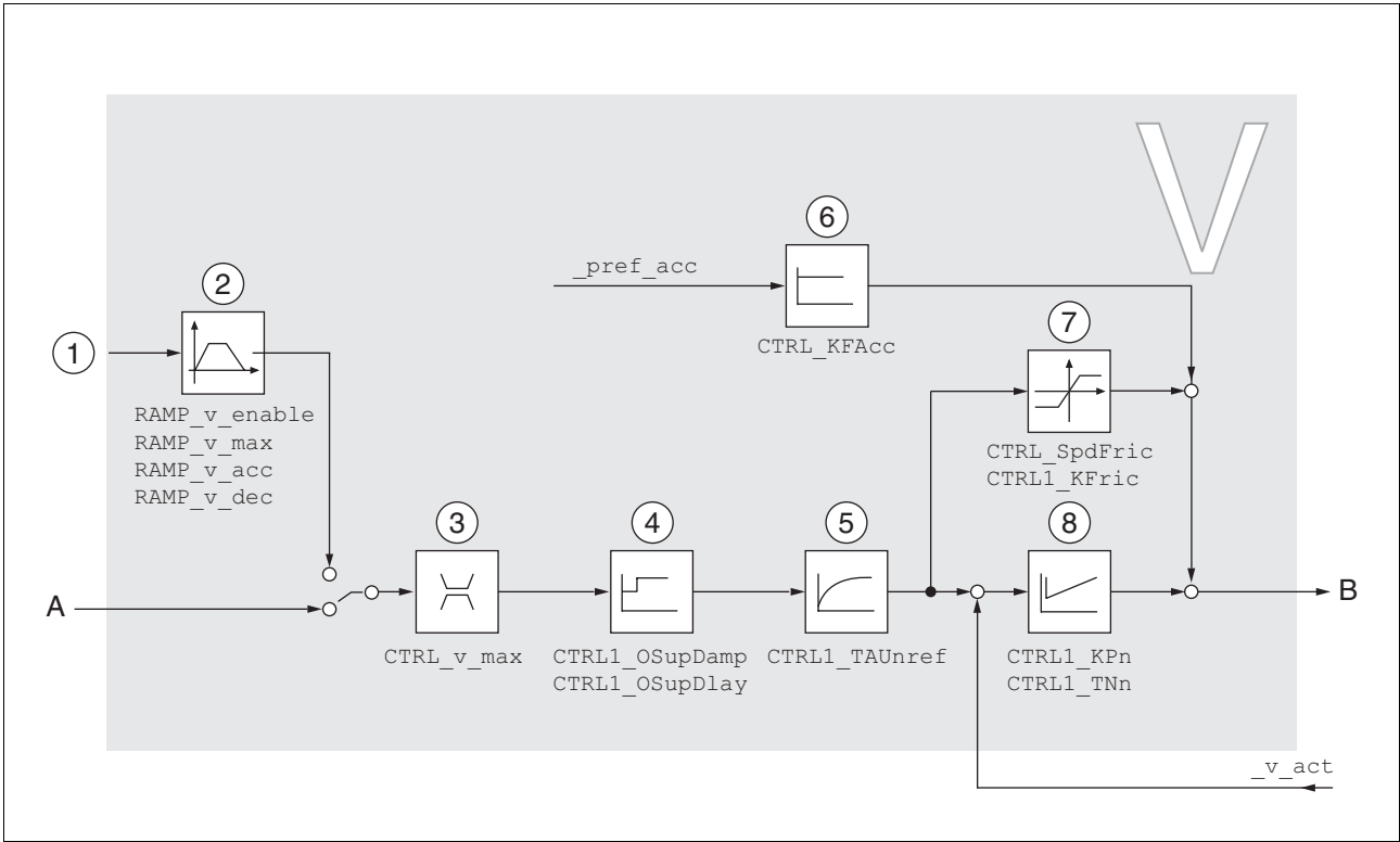
图 8.22 转速控制器
