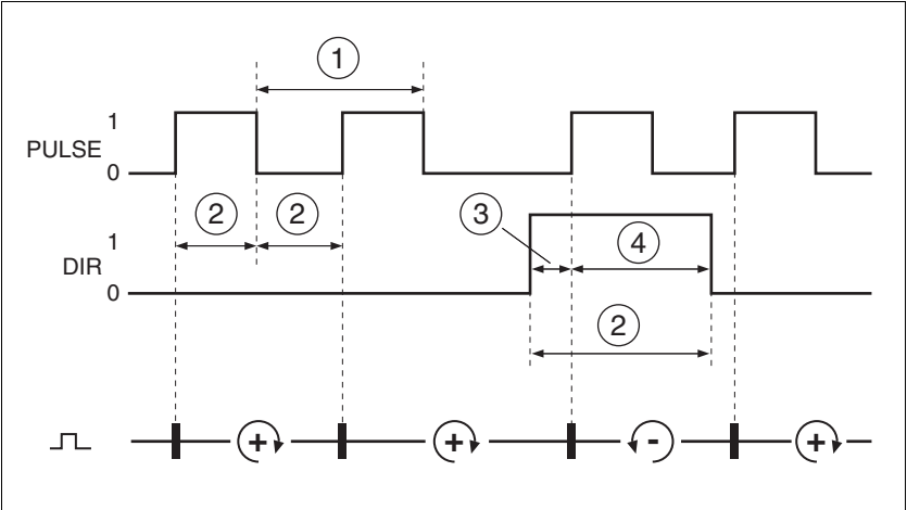
图 3.7 时间图和脉冲 / 方向信号
