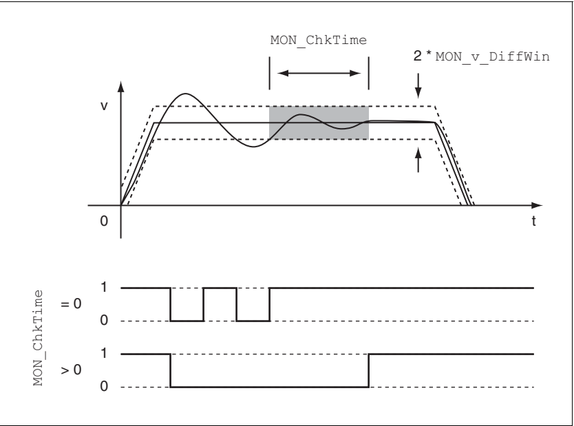
图 8.36 速度偏差窗口
