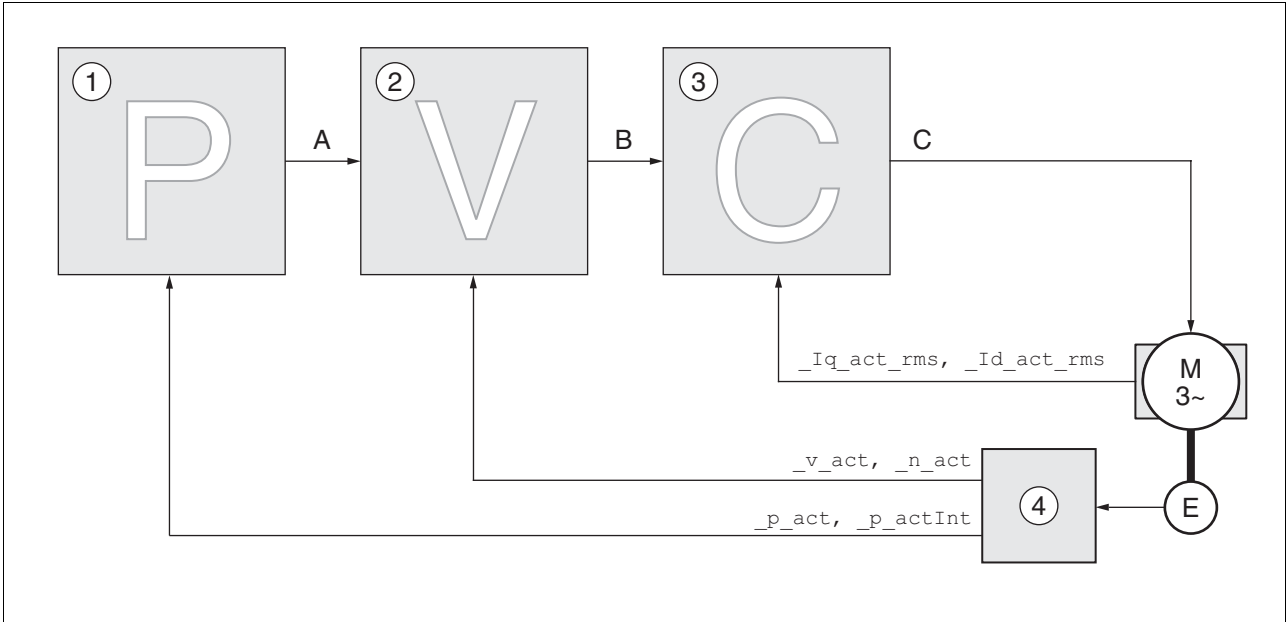
图 8.20 控制器结构概况
