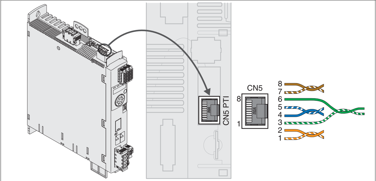
图 6.13 连续脉冲输入（PTI）接线图 5 V
