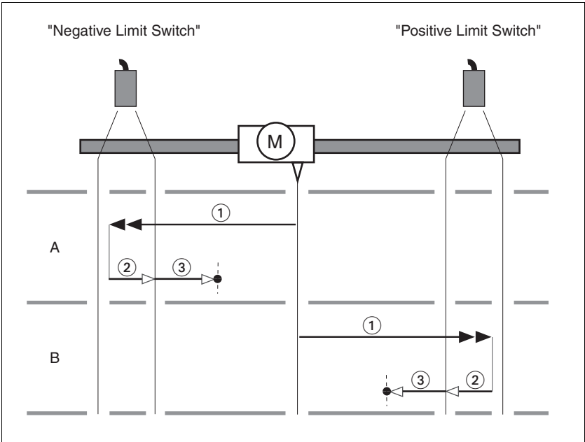
图 8.11 朝向限位开关的基准点定位运行
