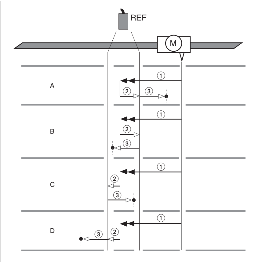
图 8.13 沿负方向朝向基准开关的基准点定位运行
