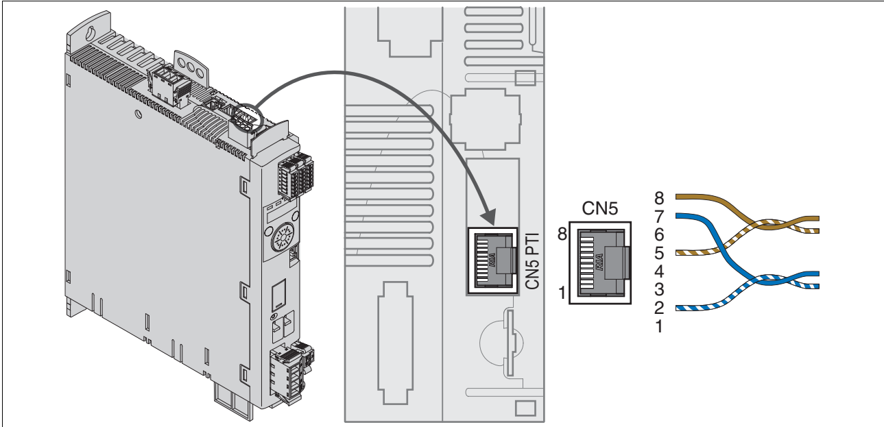
图 6.14 连续脉冲输入（PTI）接线图 24 V
