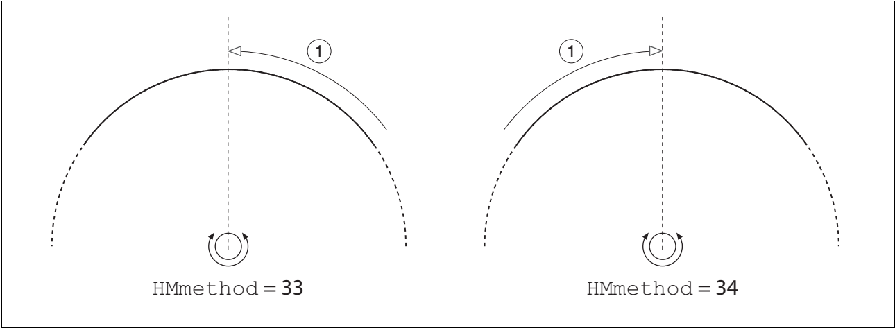
图 8.14 朝向标志脉冲的基准点定位运行
