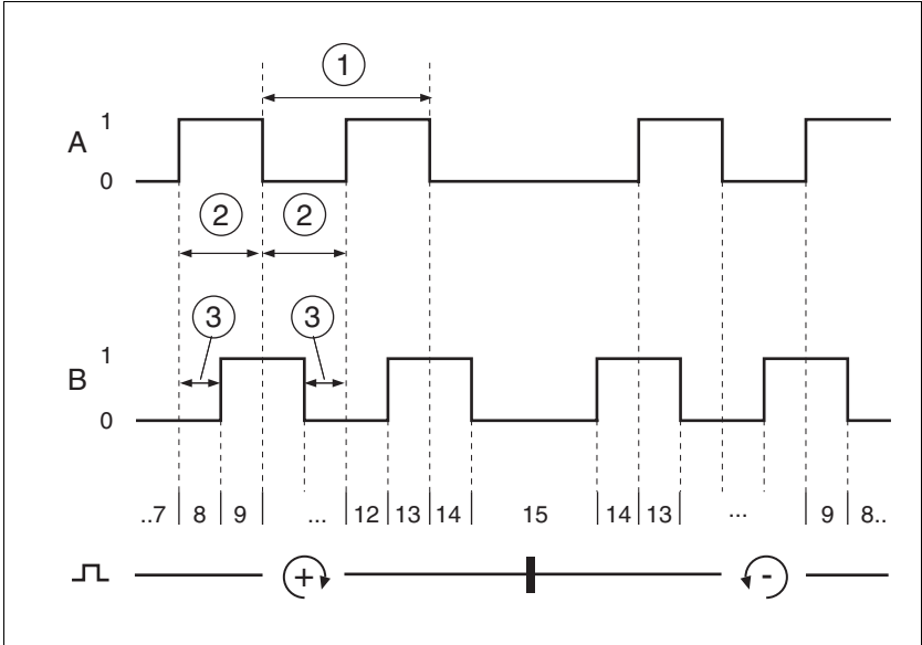
图 3.8 时间图 和 A/B 信号，向前计数，后退计数
