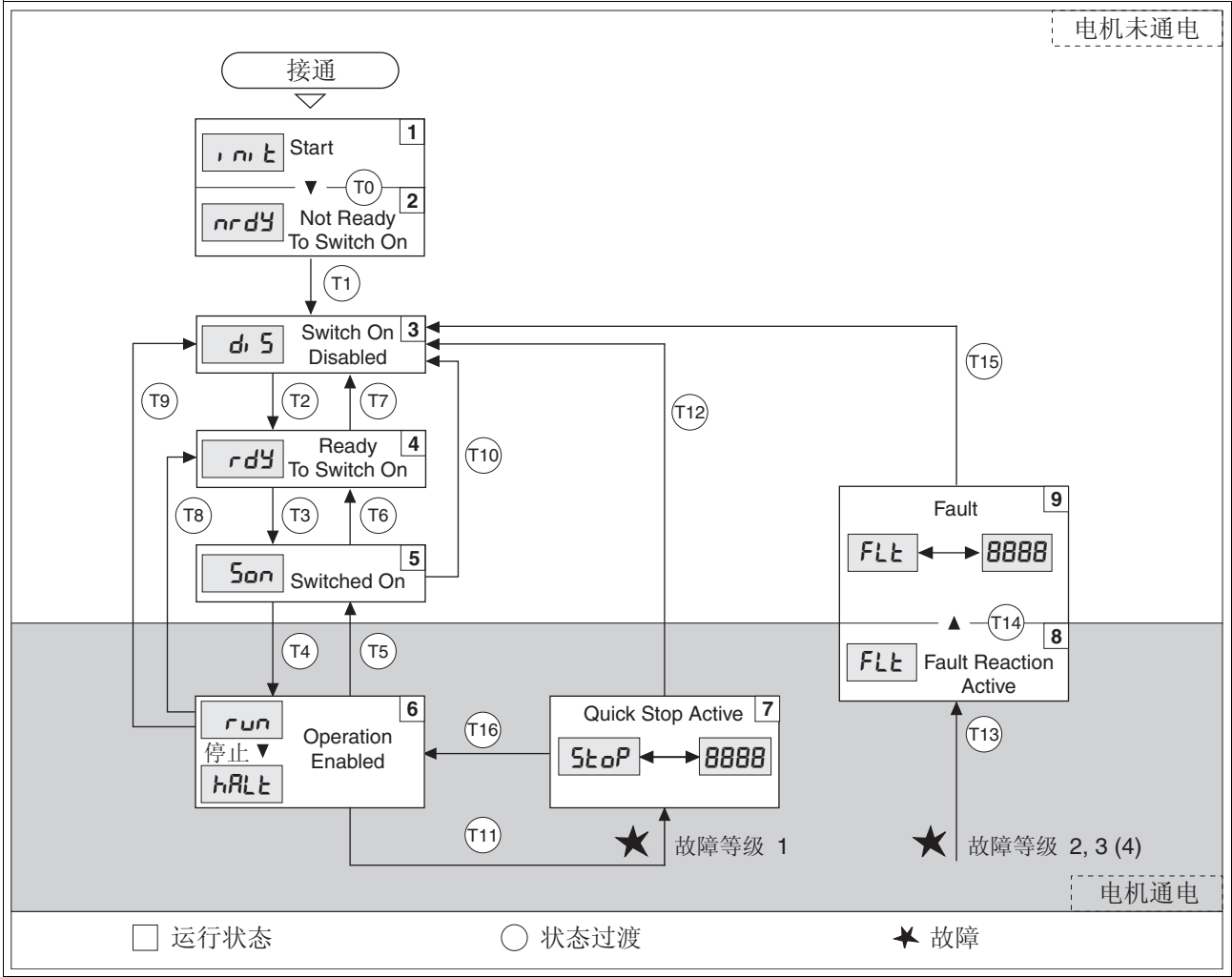
图 7.5 状态图
