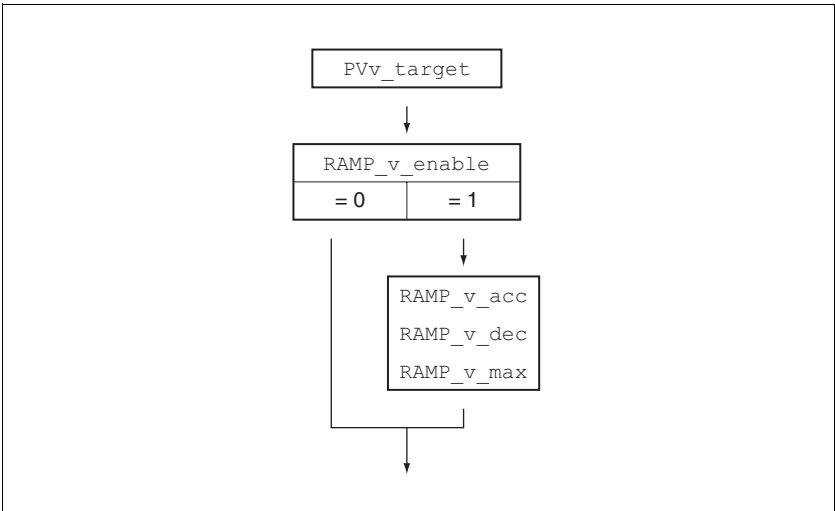
图 8.8 可设置参数的概况
