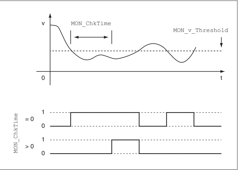
图 8.37 速度阈值
