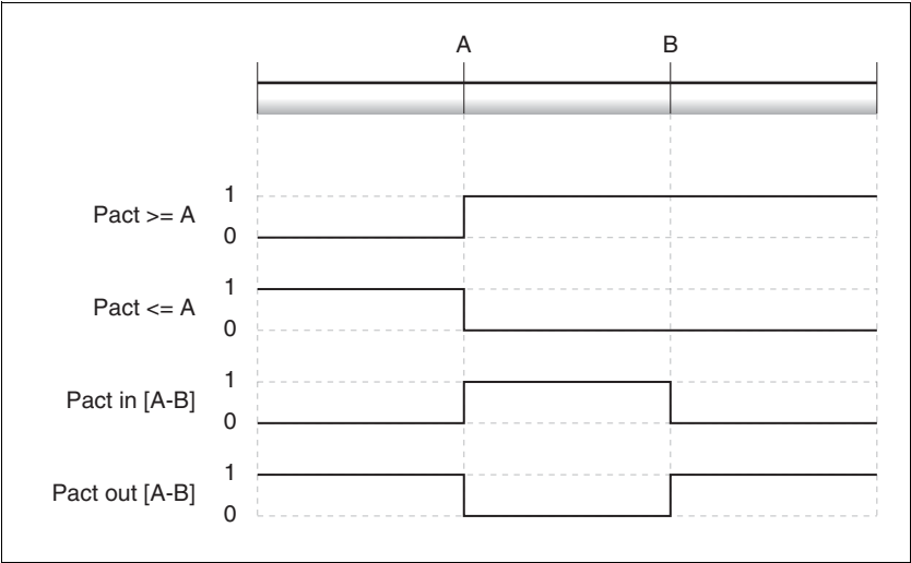
图 8.34 位置寄存器
