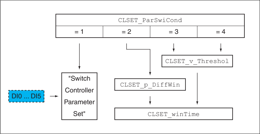
图 8.24 切换控制器参数组的参数
