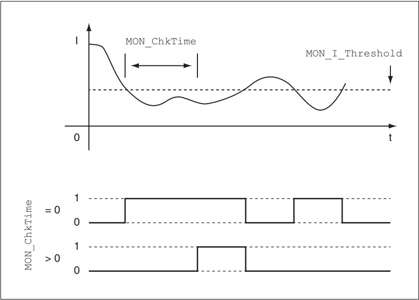
图 8.38 电流阈值
