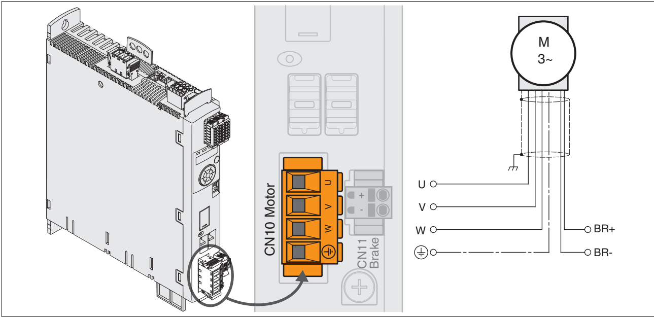
图 6.4 带止动闸的电机接线图
