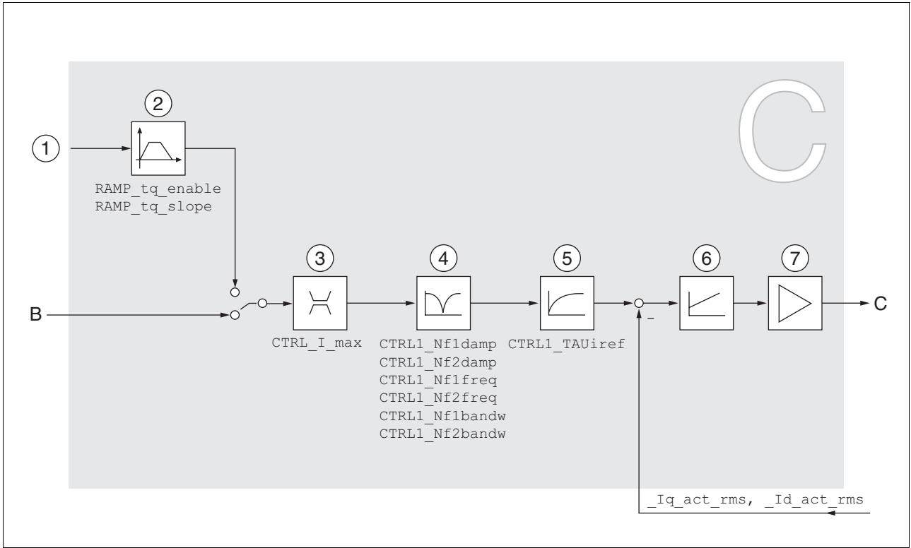
图 8.23 电流控制器
