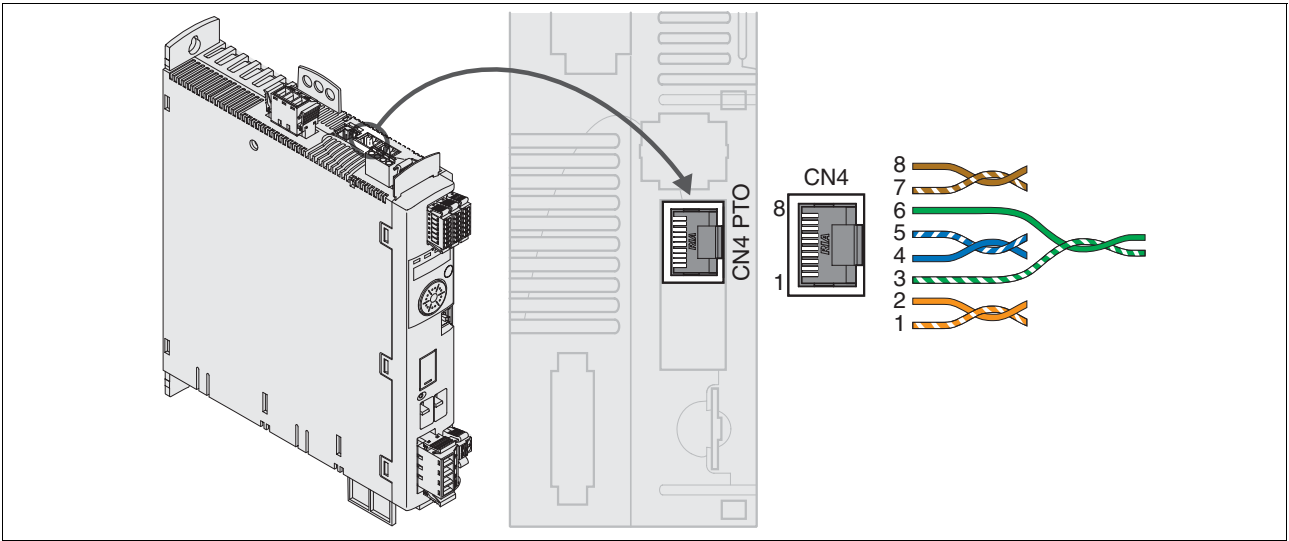
图 6. 12 连续脉冲输出（PT0）接线图
