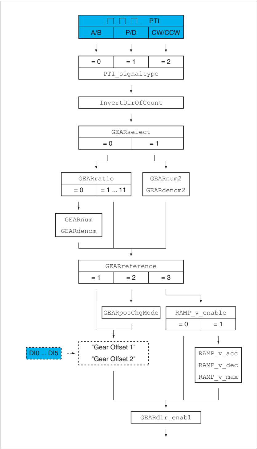
图 8.6 可设置参数的概况
