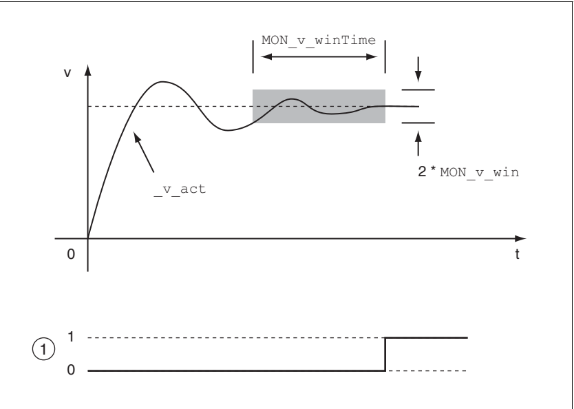
图 8.32 速度窗口
