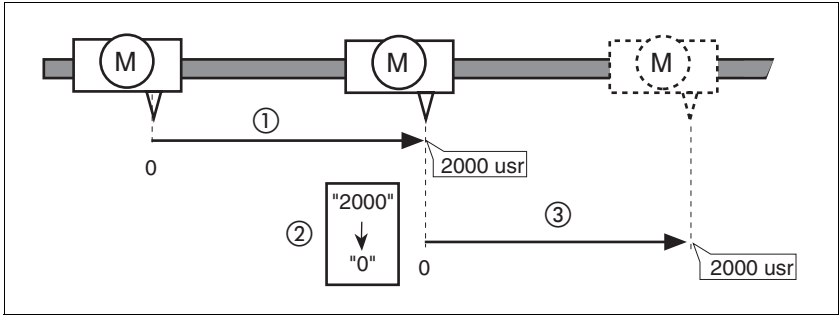
图 8.15 使用尺寸设定以 4000 usr 单位进行定位
