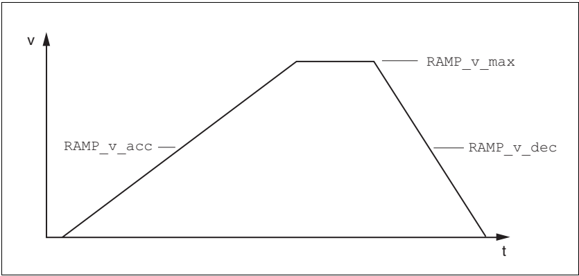
图 8.27 斜坡陡度
