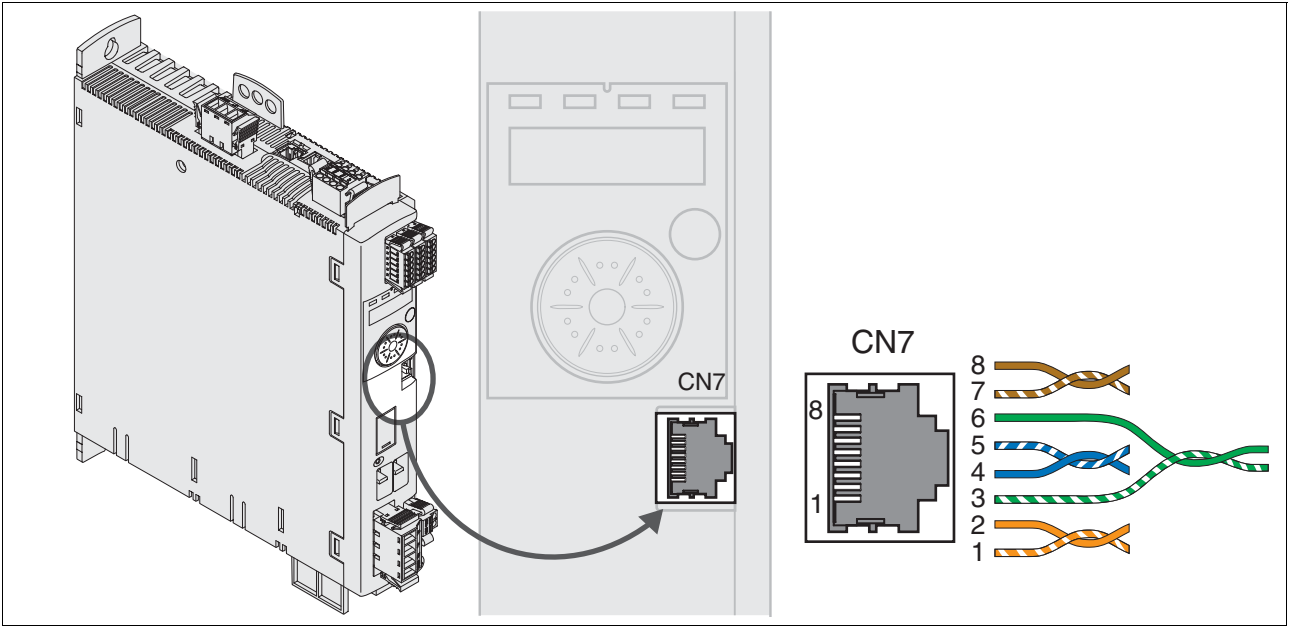
图 6.17 装有调试软件的 PC 接线图
