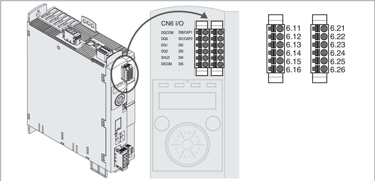
图 6.16 数字输入 / 输出接线图
