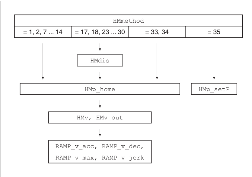
图 8.10 可设置参数的概况
