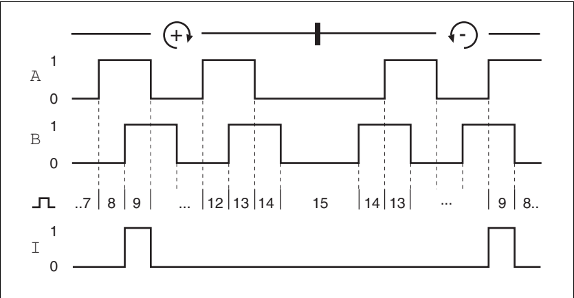
图 3.5 A、B 和标志脉冲信号时序图, 正向与反向计数
