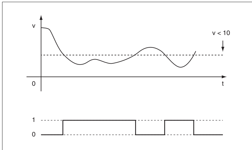
图 8.30 电机停止
