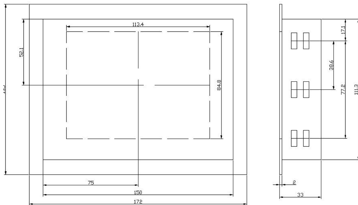
LR056VR/A系列液晶显示器前嵌式金属壳安装尺寸图
