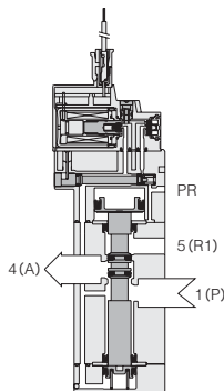
G180E1-11 不通电时
