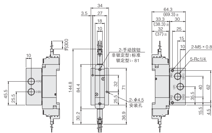
GA180_4E
