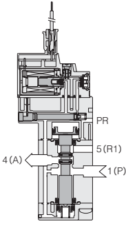
G110E1-11 不通电时
