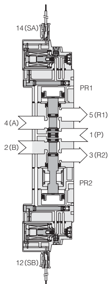
G183-4E2-13
