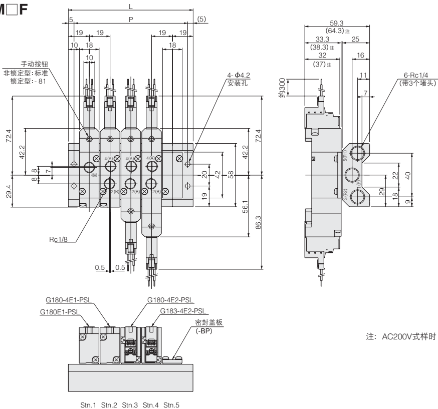
汇流板尺寸图 2 · 3 · 5通混合安装用 (mm)
