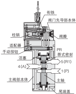
G110E1 不通电时
