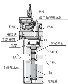
G180E1 不通电时
