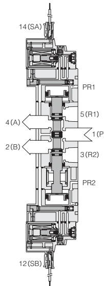
G183-4E2-14
