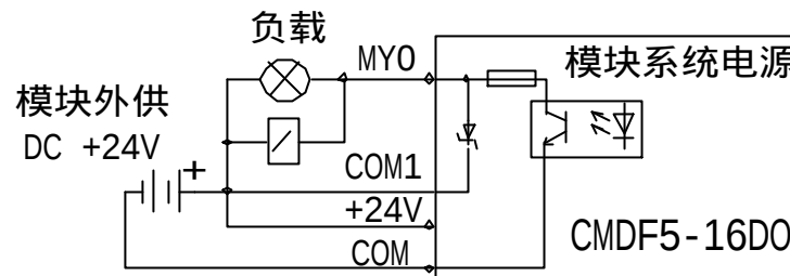
图 6 漏输出（NPN）电原理框图
