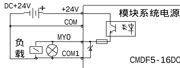
图 7 源输出（PNP）电原理框图
