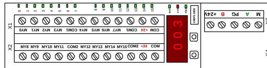
(图 8) CMDF1-16DO 端子示意图
