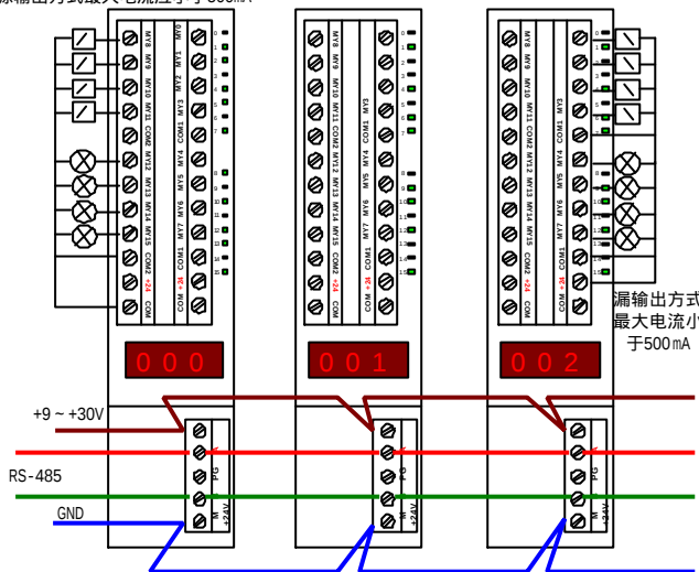
(图 10) CMDF1-16DO 接线参考示意图
