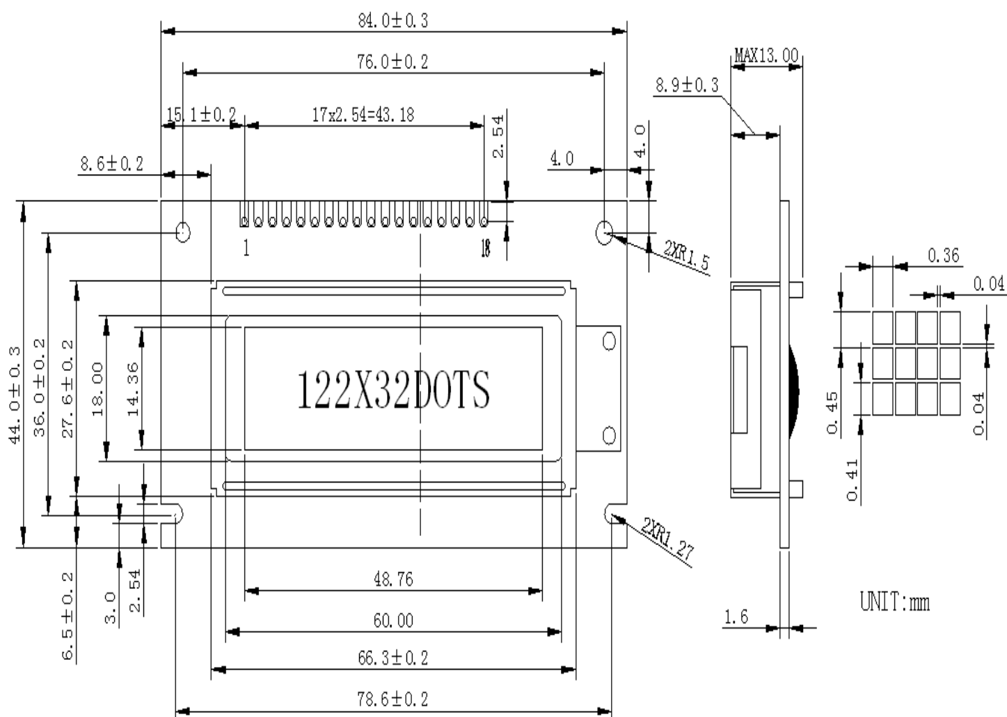
JD12232D2 尺寸图
