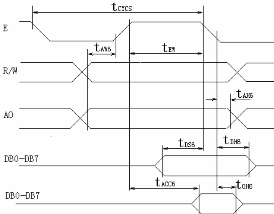
时序 1
