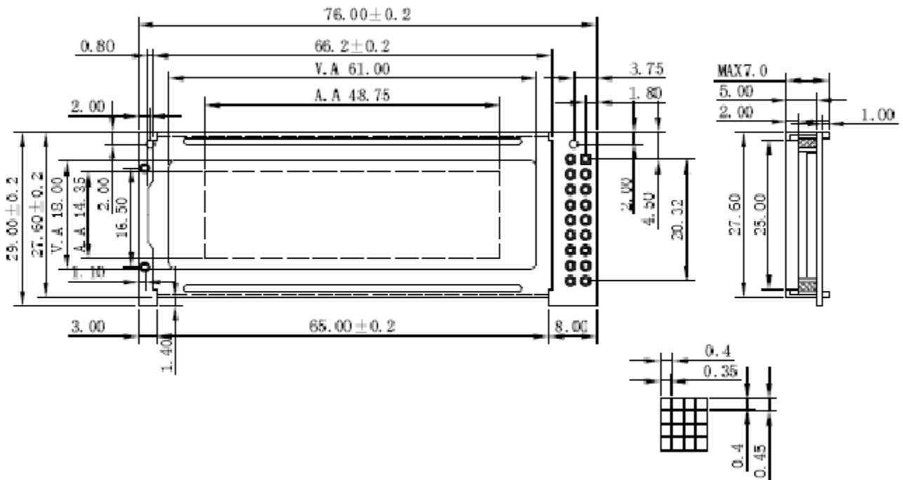
JD12232A3 尺寸图
