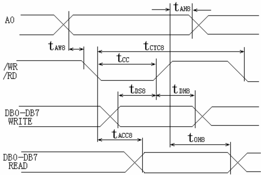
时序 2
