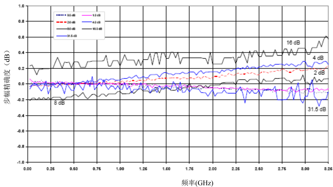
典型 AT4610 步幅精度
