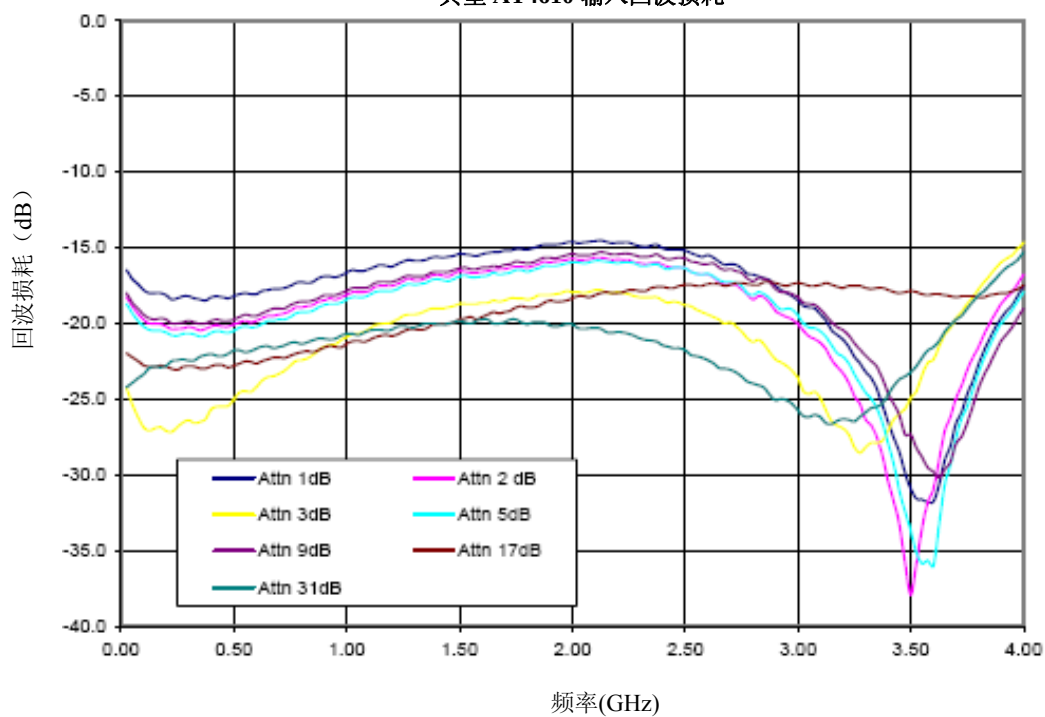
典型 AT4610 输入回波损耗
