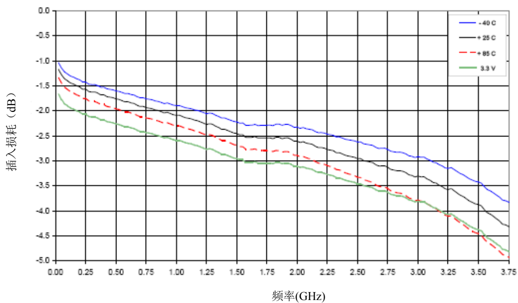
典型 AT4610 参考插入损耗
