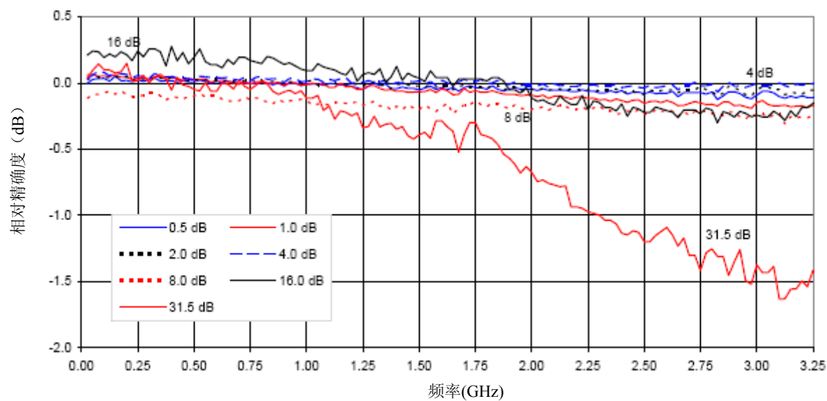
典型 AT4610 相对精度
