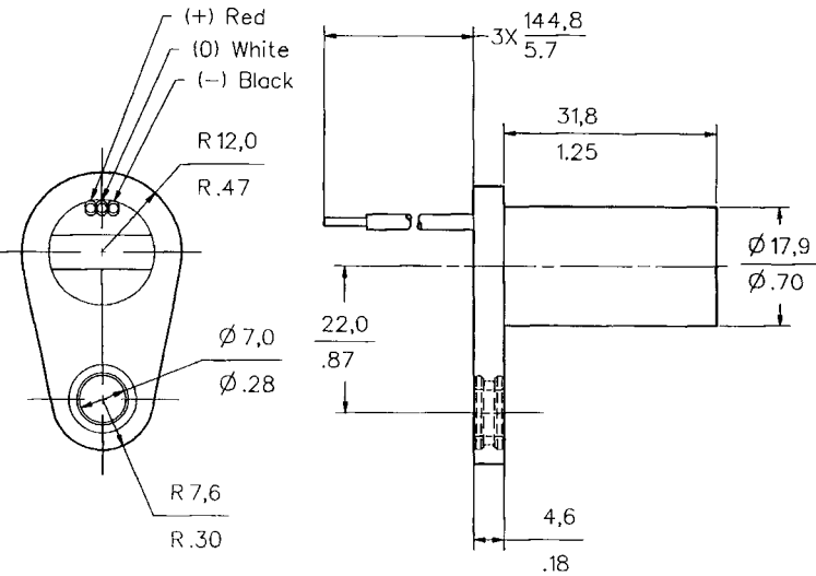
安装尺寸 (仅供参考)
