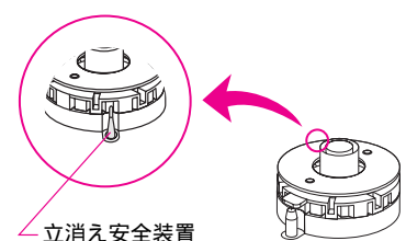
後方から見た図 (例) 標準バーナー
