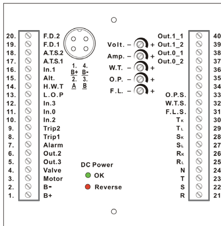
圖 2 GTR-80 背板
