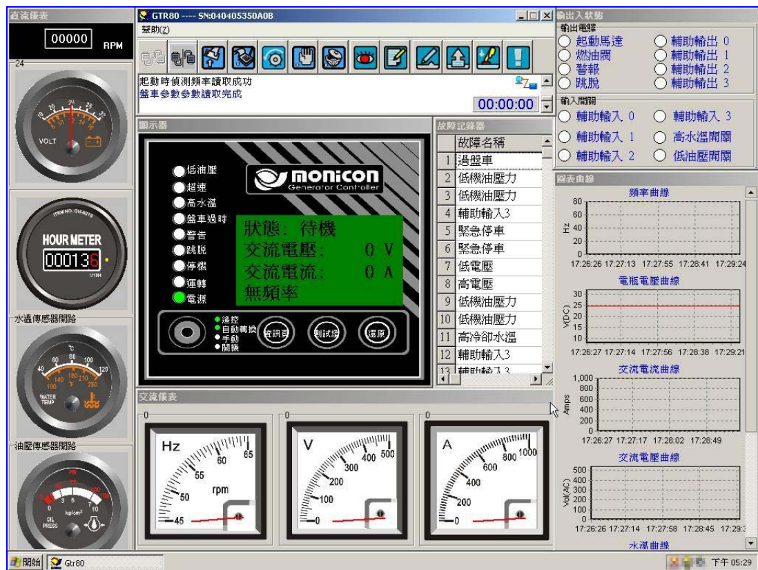
圖 17 監控畫面(本軟體畫面解析度以 1024X768 為主。)
