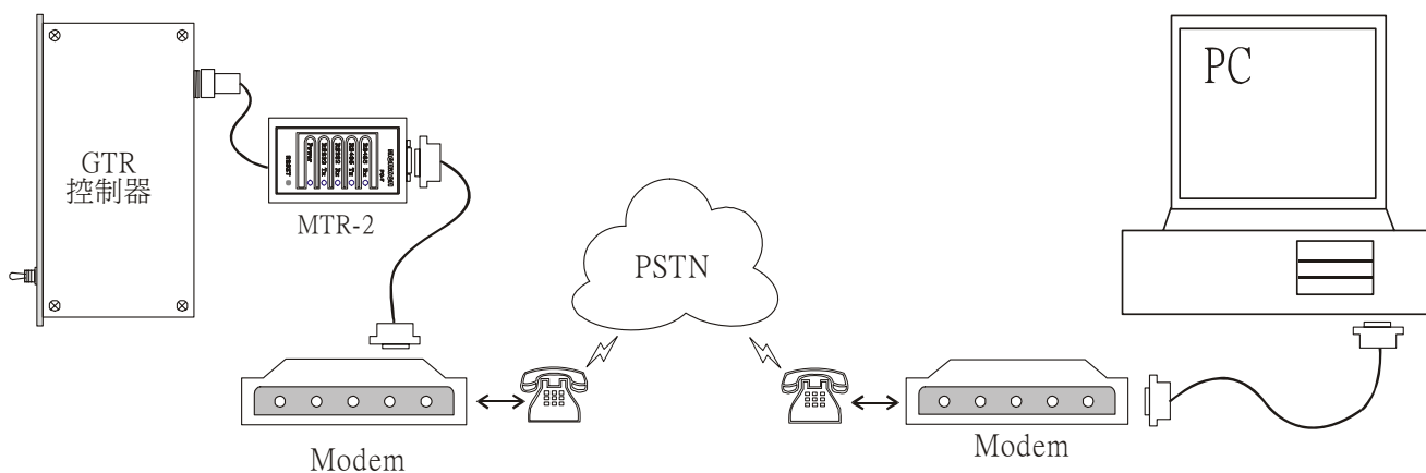
圖 6 遠端連線示意圖
