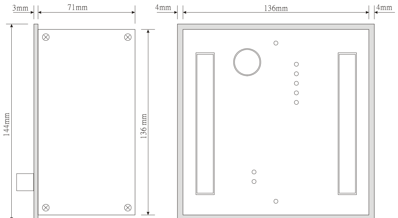
圖 3 GTR80 控制器側視圖及背視圖之相關尺寸
