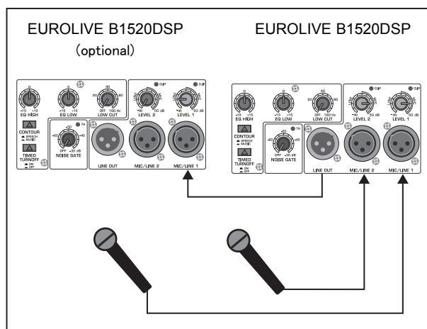
图 3.1: 麦克风连接
