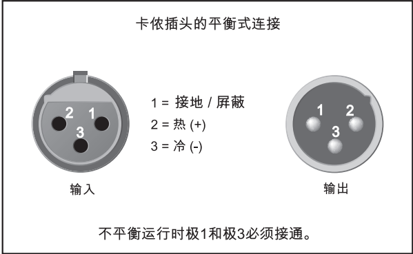
图 4.1: XLR 插头
