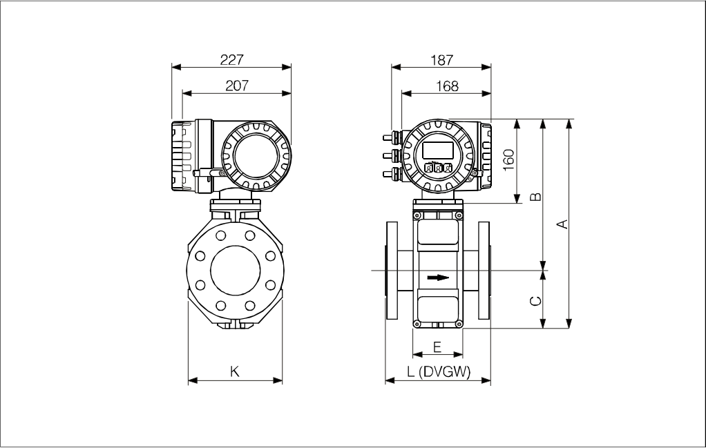
Promag W / DN ≤ 300 (一体化型)
