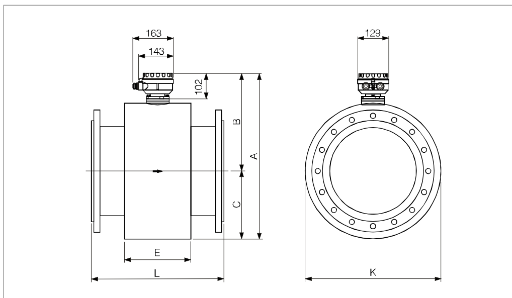
Promag W / DN ≥ 350 (分离型)
