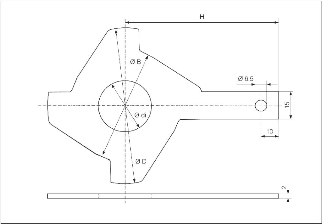
接地环（DN 25...300）
