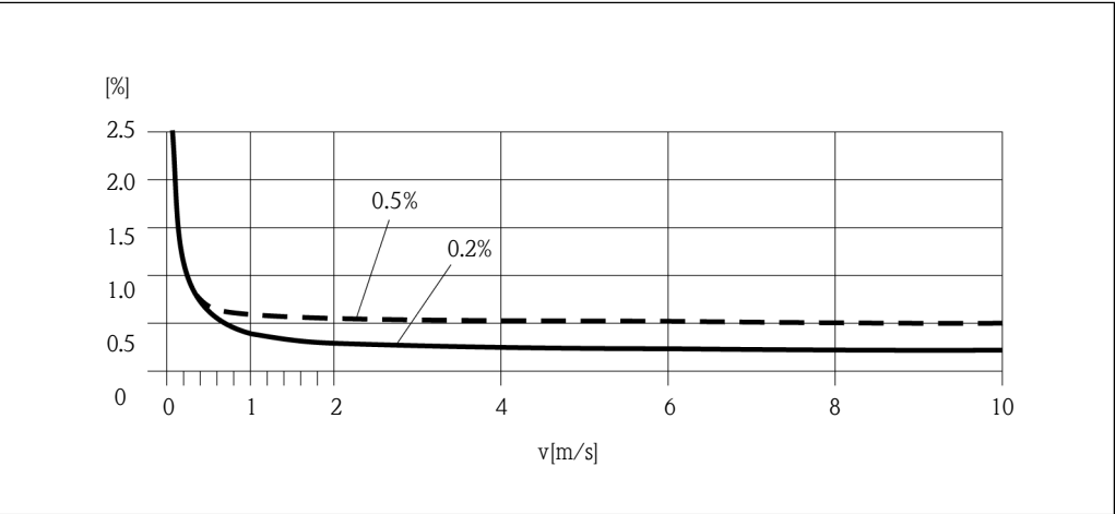
最大测量误差：% o.r.
