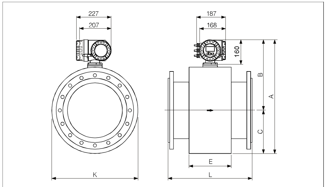
Promag W / DN ≥ 350 (一体化型)
