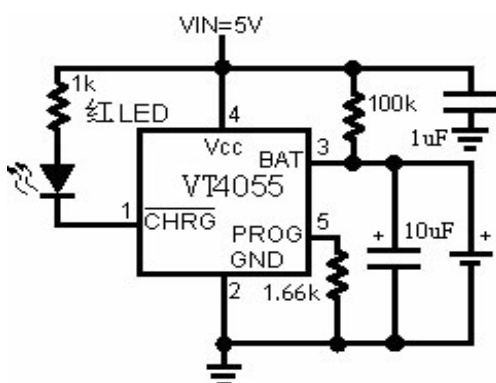
无电池不闪灯单节锂电池充电器 (无电池红灯灭, 不影响其他状态指示)
