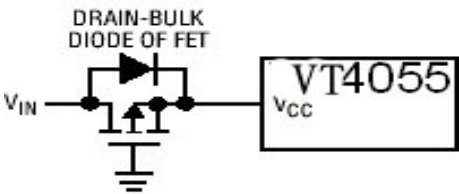
图 5：低损耗输入反向极性保护
