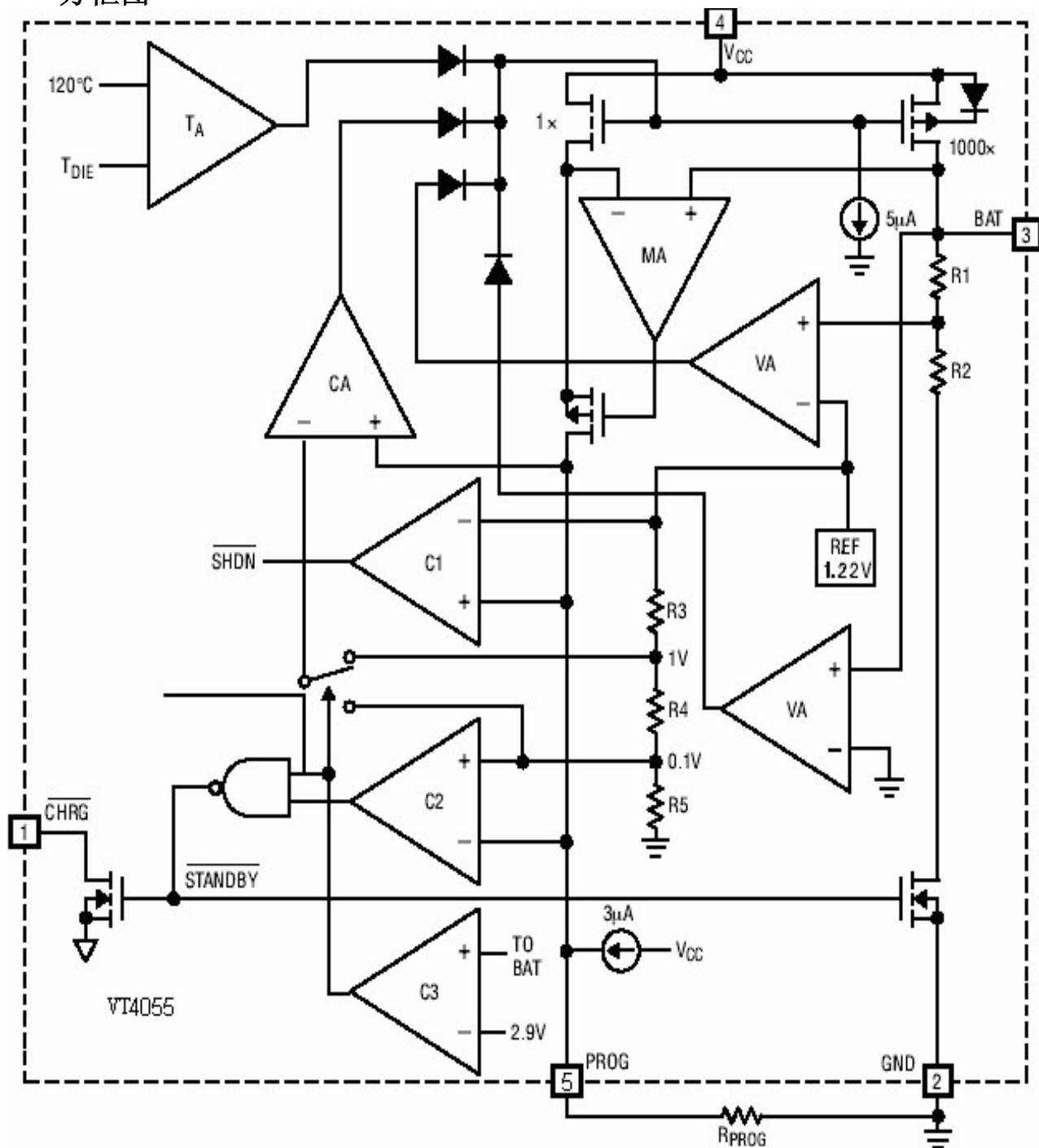
方框图
