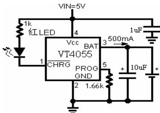
全功能单节锂电池充电器 (无电池状态红灯闪烁)
