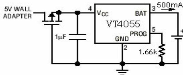
具有输入反向极性保护的充电器
