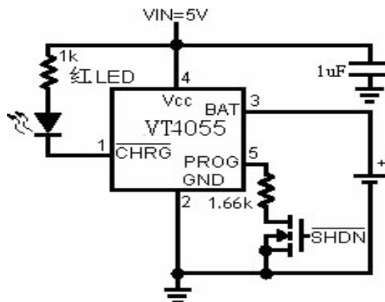
图 1：可信号控制充电电路
