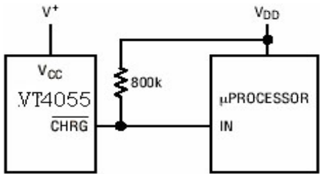
图 4：采用一个微处理器来确定 CHRG 引脚状态
