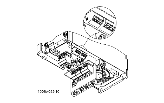
继电器连接端子。
