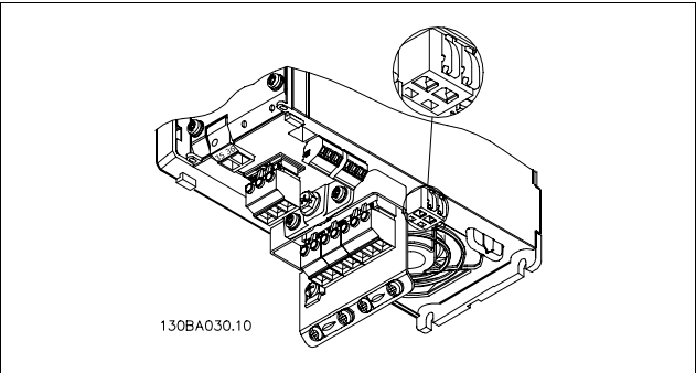
用于 LC 滤波器选件的直流回路反馈的端子。
