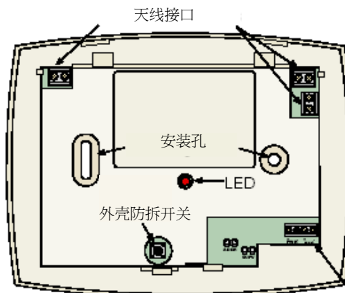
电源和总线接口
