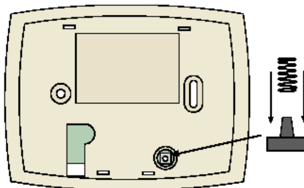
接收器的后部面板
