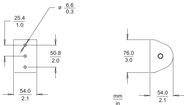
可调节安装头的外形尺寸
