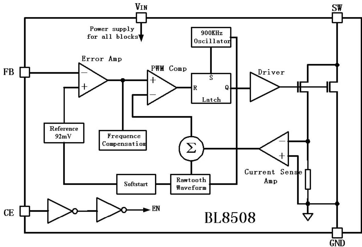
系统框图:
