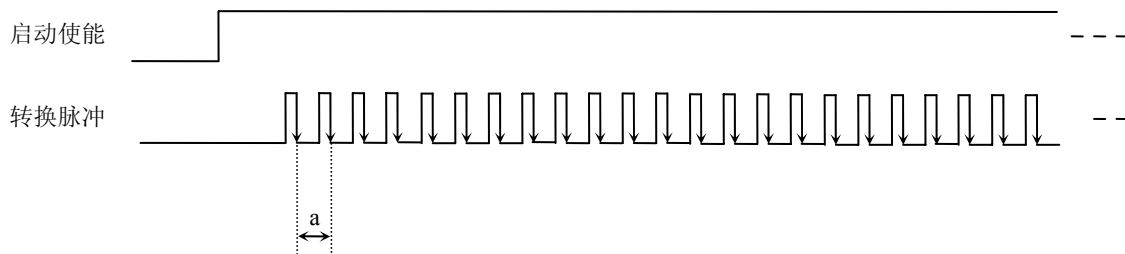
图 7.2 内时钟模式下的连续采集
