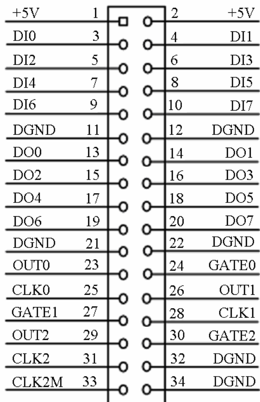
关于 34 芯插头 P1 的管脚定义（TTL 开关量输入/输出）（表格方式）
