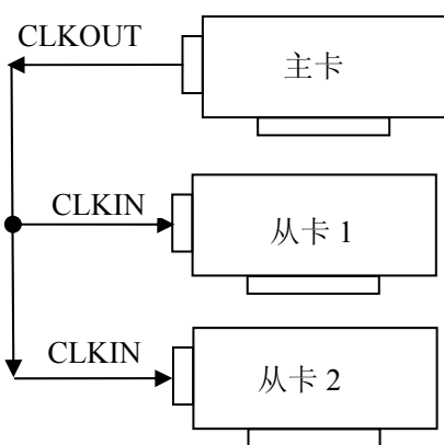
多卡的级联方法
