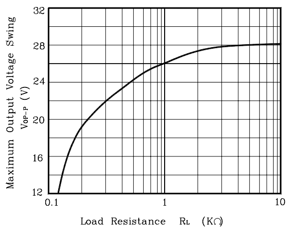
Fig. 5 V_{OP-P} - R_L
