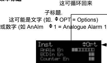
图 3-2: 参数菜单标题
