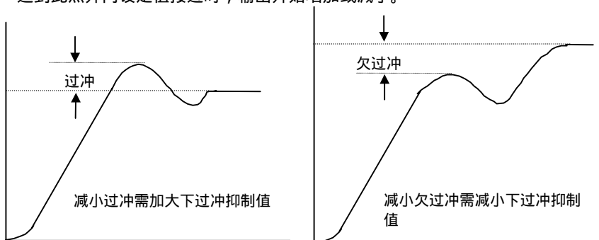
图 20-3: 低过冲抑制
