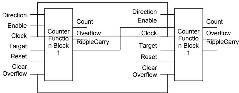
图 14-2: 计数器串联
