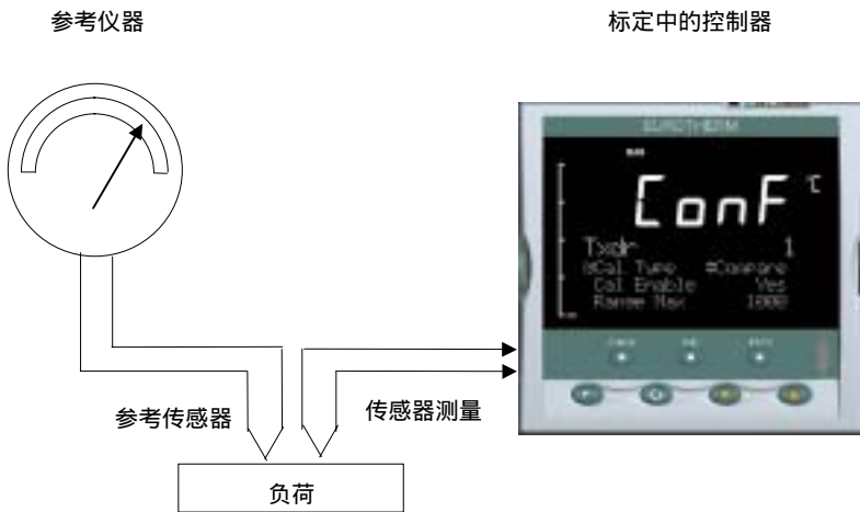
图 23-4: 比较校准
