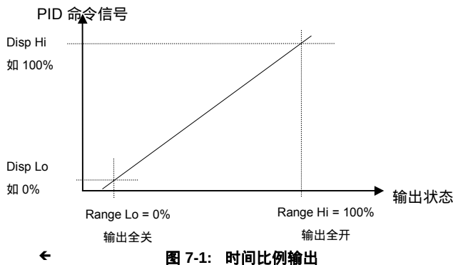
图 7-1: 时间比例输出
