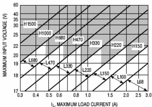
LM2576-15
