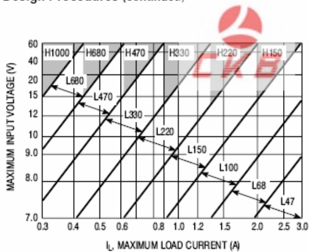
LM2576-5
