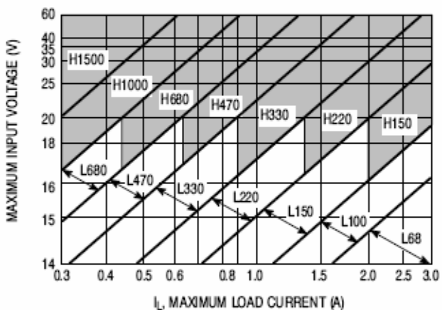
LM2576-12
