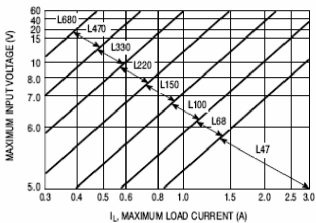
LM2576-3.3
