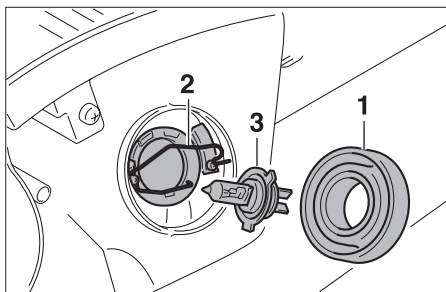
1. 防塵套 2. 前燈固定支架 3. 前燈燈泡
