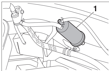
1. 活性碳罐
