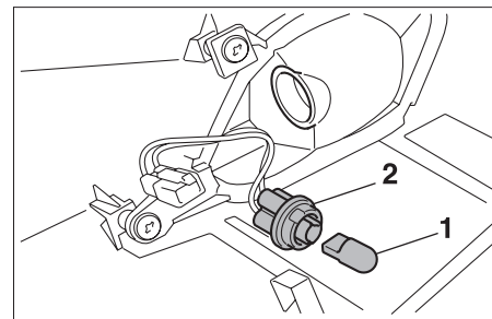
1. 前方向燈燈泡 2. 前方向燈燈泡固定座
