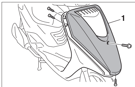
1. 上前擋泥蓋(螺絲x6)
