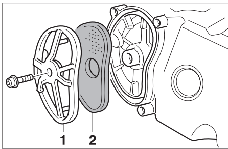
1. 濾網固定座 2. 濾清器濾網
