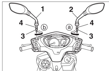
1. 左後視鏡 2. 右後視鏡 3. 固定螺栓 4. 可傾倒部份固定螺帽
