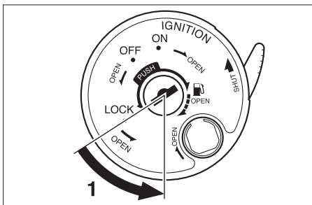
1. 座墊開啟 (在LOCK位置)
