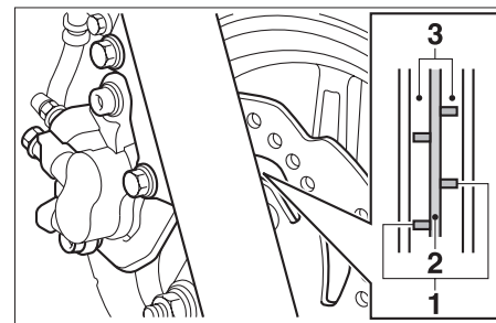
1. 磨耗指示器 2. 煞車圓盤
