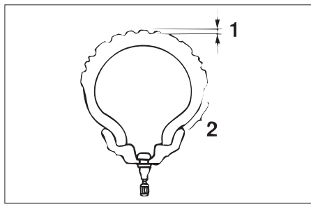
1. 胎紋 2. 胎壁
