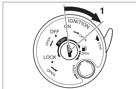
1. 座墊開啟 (在ON位置)
