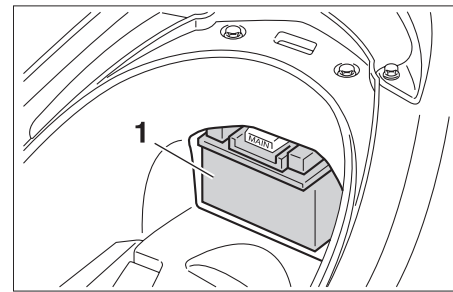
1. 電瓶
