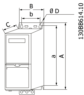
外形尺寸
