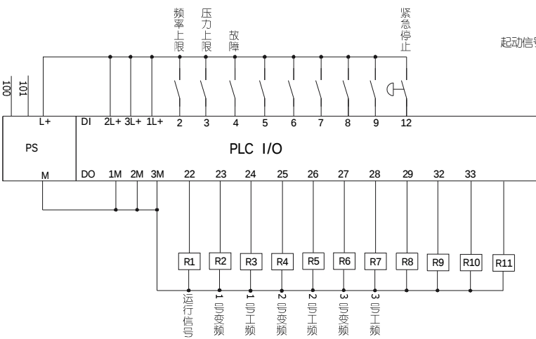
PLC接线图
