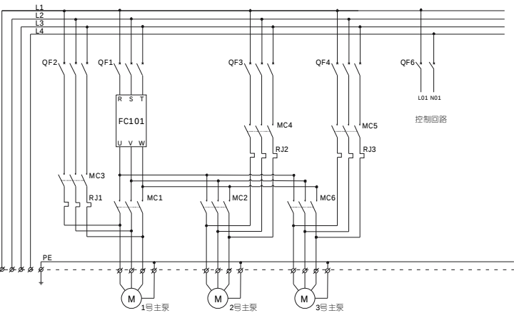
主回路图
