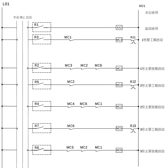
控制回路图
