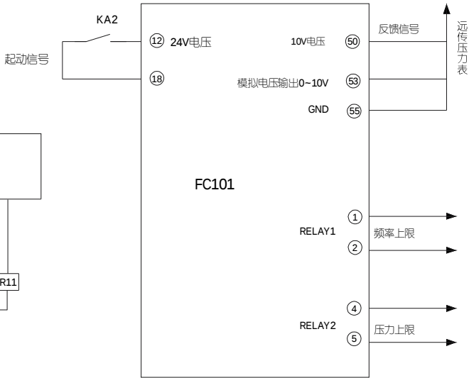
FC101接线图
