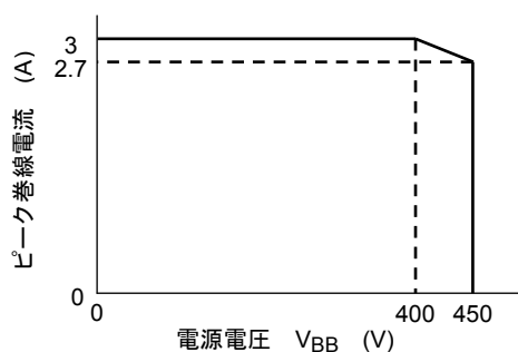
図 1: T_j = 135 \text{ }^{\circ}\text{C} の安全動作領域
