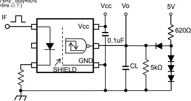
図8 伝達遅延時間測定回路、波形
