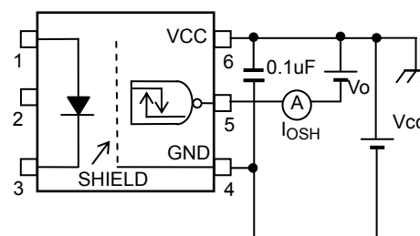
図6 I_{OSH} 測定回路
