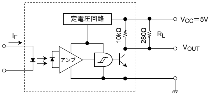
TLP1006A(F)
