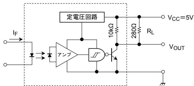
TLP1007A(F)
