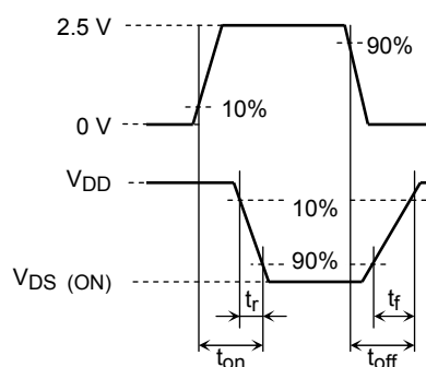
(c) 出力波形
