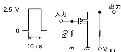
(a) 測定回路
