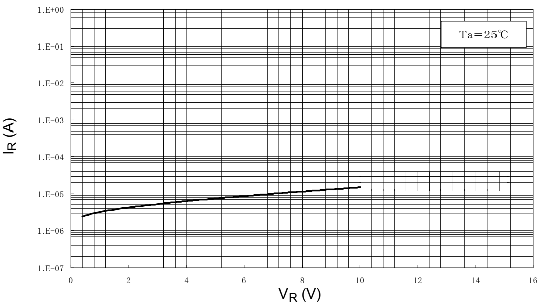
I_R - V_R
