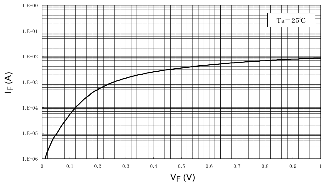
I_F - V_F
