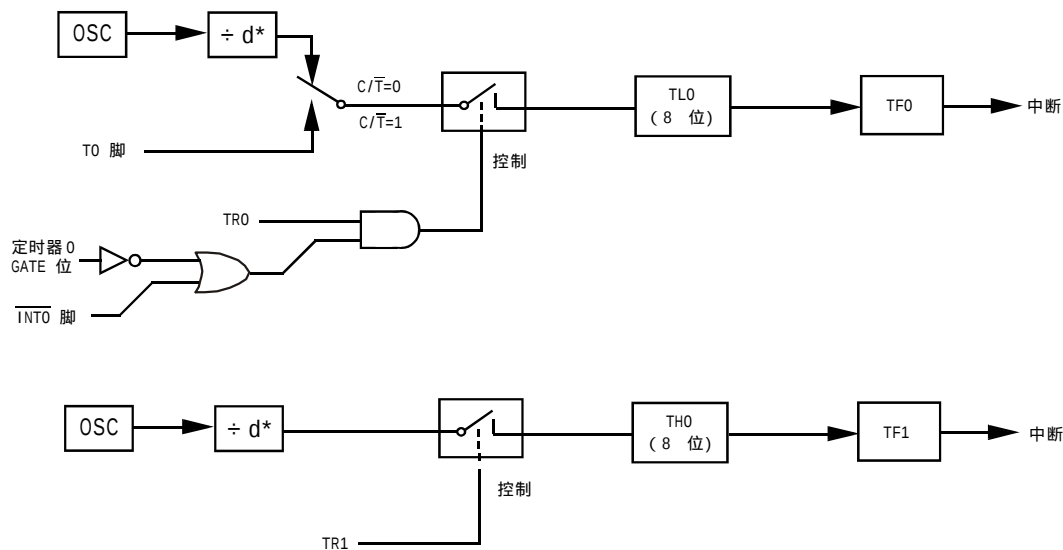
图 定时 / 计数器 0 的模式 3 : 两个 8 位计数器
