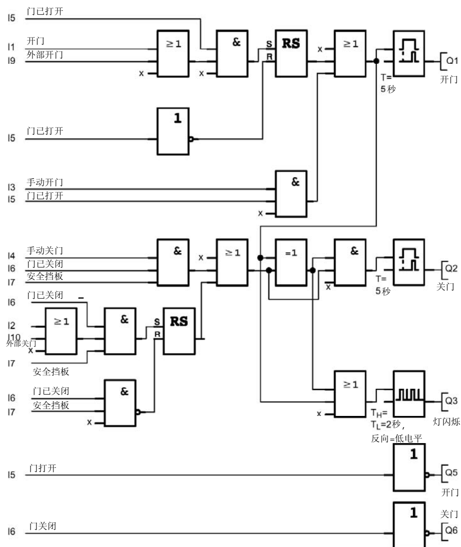
使用 LOGO! 方案的功能块图
