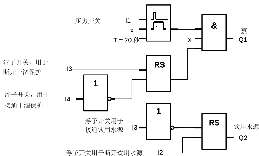
使用 LOGO! 的功能块图
