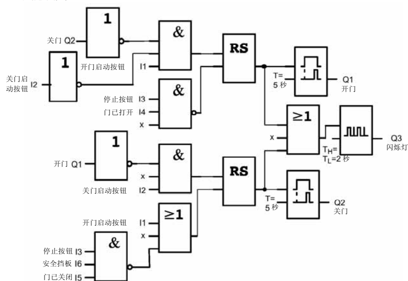
使用 LOGO! 的功能块图
