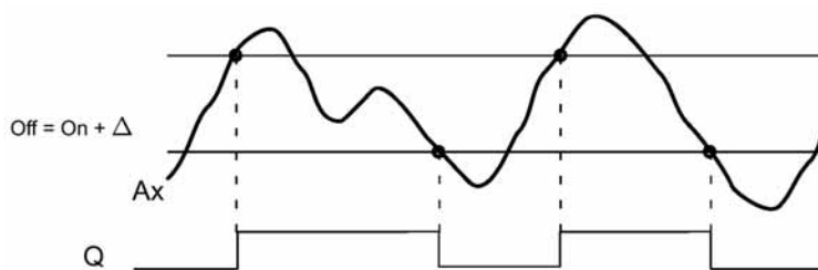
时序图B：偏差 \Delta 为正值时的时序图
