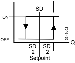
正向动作顺序 (应用编号.：80-89)
