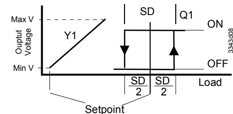
2个均为正向动作 (不关联控制回路) (应用编号：70-79)
