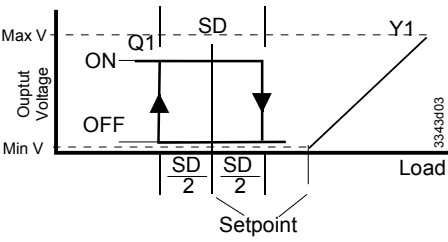
反向和正向动作顺序 (应用编号.：40-49)
