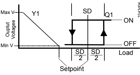
反向和正向动作顺序 (应用编号.：50-59)
