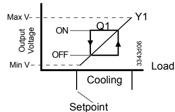
2 个均为正向动作顺序 (关联控制回路) (应用编号：60-69)
