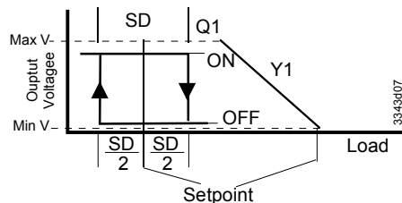
2个均为反向动作 (不关联控制回路) (应用编号：30-39)
