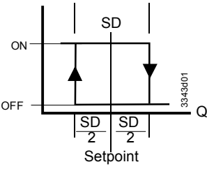
反向动作顺序 (应用编号：10-19)
