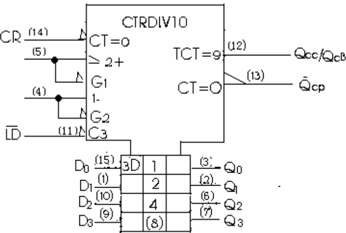
逻辑符号
