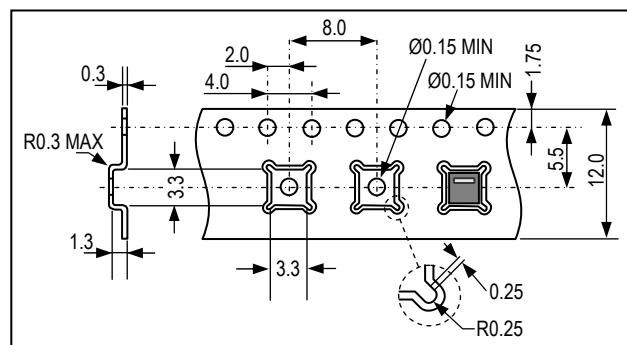
图 22 包装卷带和传感器定位图
