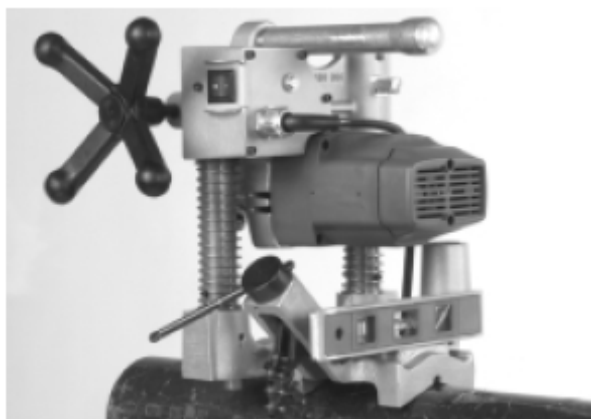
图17 — 用水平仪来叫准位置
