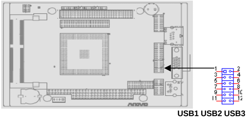
USB引脚定义
