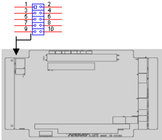
网络插针引脚信号
