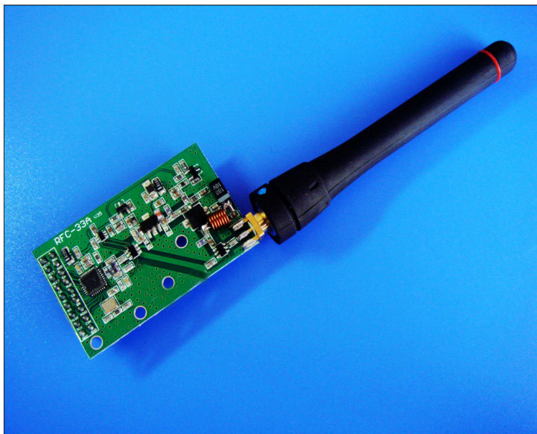
RFC-33A (尺寸: 51mm X 31mm 板厚: 1mm)
