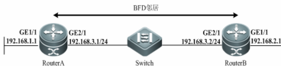
图 15 策略路由与 BFD 联动拓扑图
