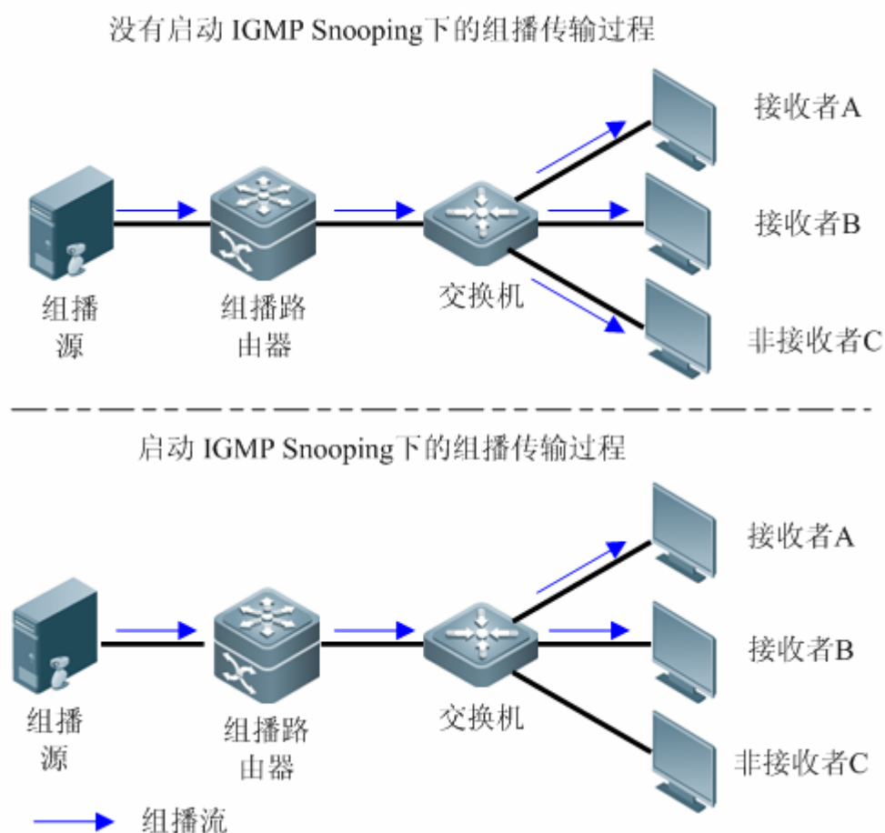
图 1-1 VLAN 上运行 IGMP Snooping 前后的对比
