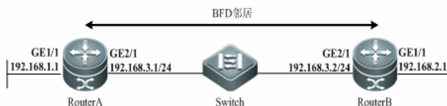
图 14 静态路由与 BFD 联动拓扑图
