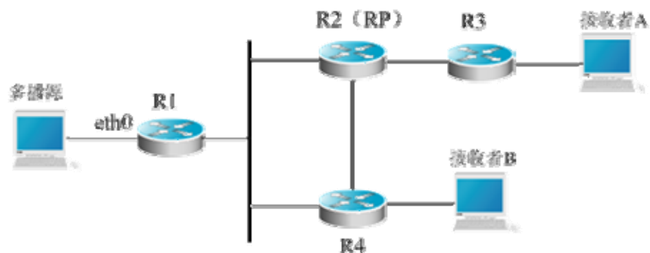
图 7 PIM-SM 配置范例拓扑结构图
