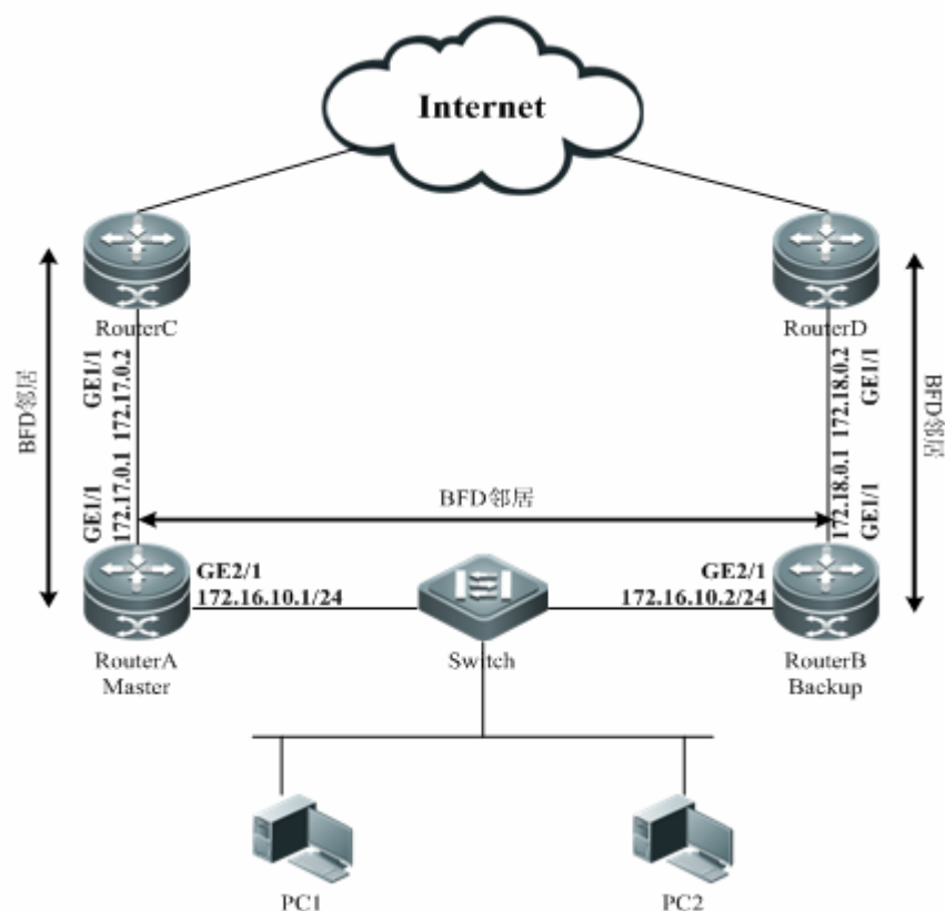
图 16 VRRP 与 BFD 联动拓扑图
