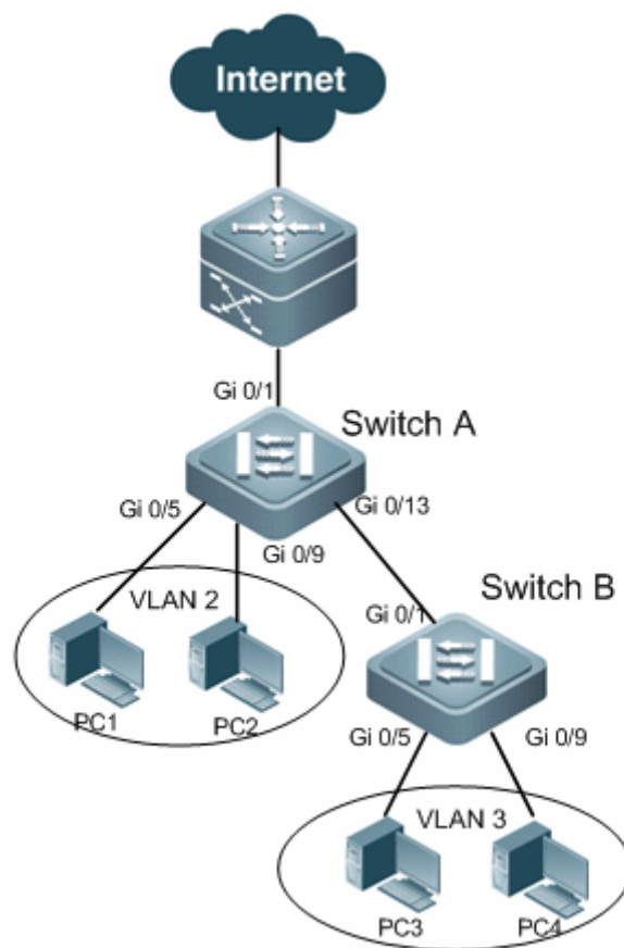
图 9 网络拓扑
