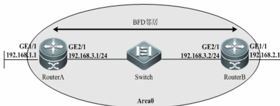
图 13 OSPF 与 BFD 联动拓扑图
