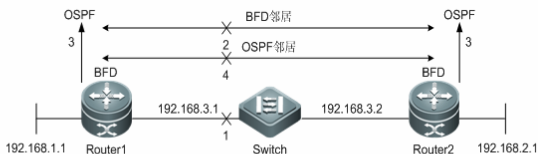
图表 4 BFD 会话检测故障处理过程
