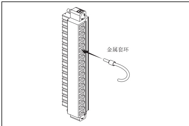
图 2 16 引脚可拆卸式螺栓端子连接器，带金属套环
