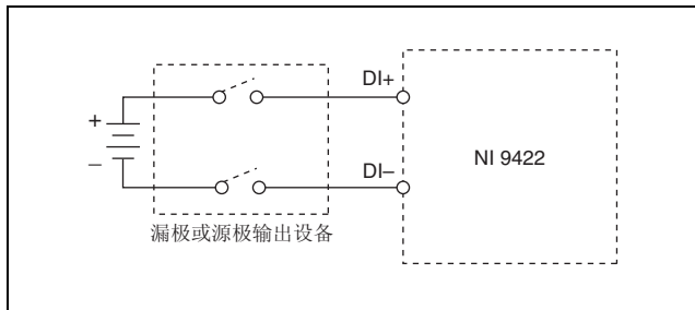
图 3 连接漏极或源极设备至 NI 9422
