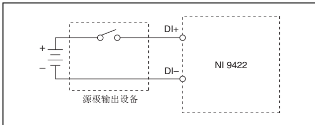
图 5 连接源极输出设备至 NI 9422
