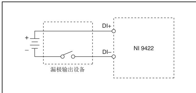
图 4 连接漏极输出设备至 NI 9422
