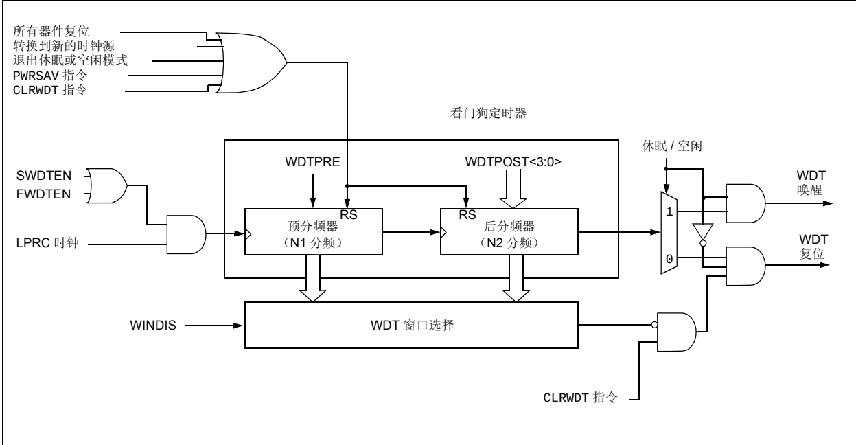
图 21-2: WDT 框图
