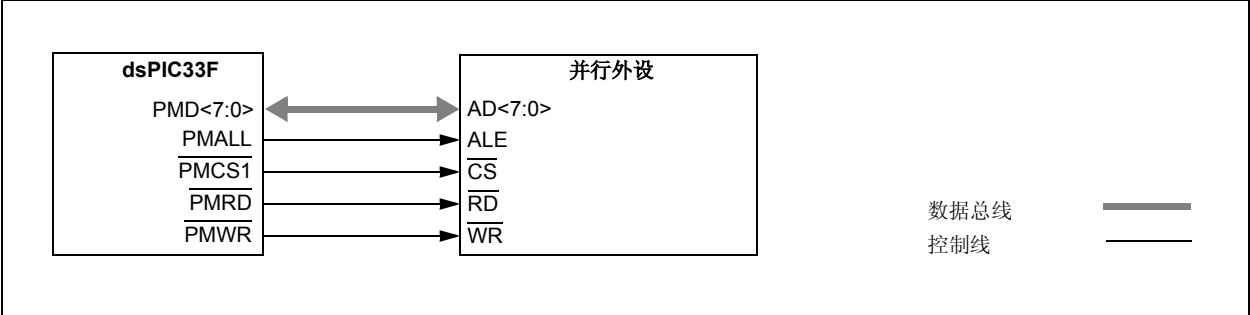
图 25-9: 8 位复用地址和数据应用示例
