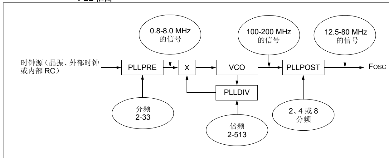
图 8-2: dsPIC33FJ32GP302/304、dsPIC33FJ64GPX02/X04 和 dsPIC33FJ128GPX02/X04 PLL 框图
