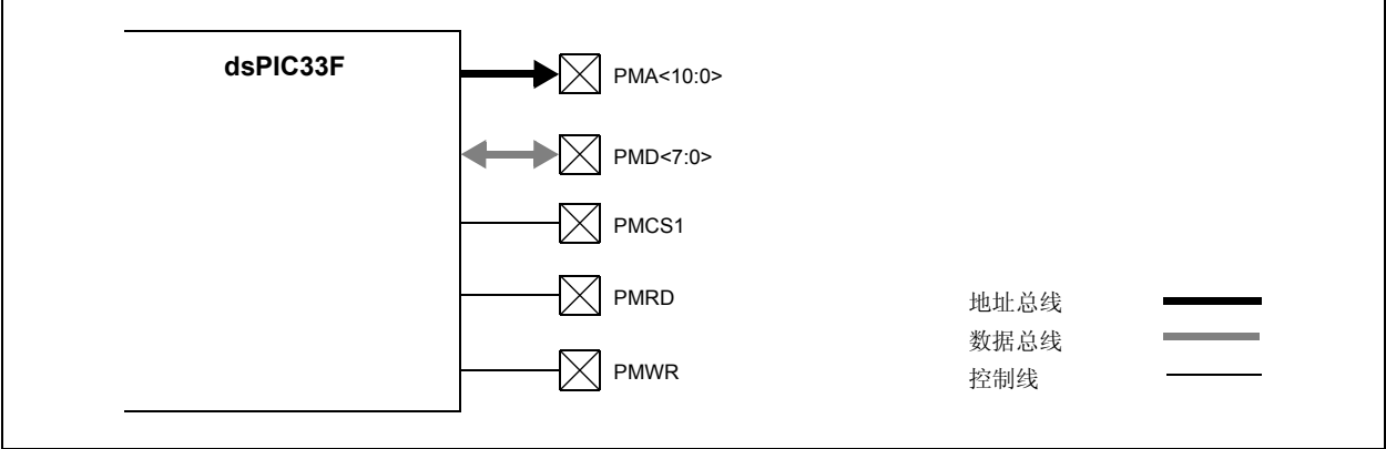
图 25-4: 主模式，未复用的寻址（独立读和写选通，单片选）
