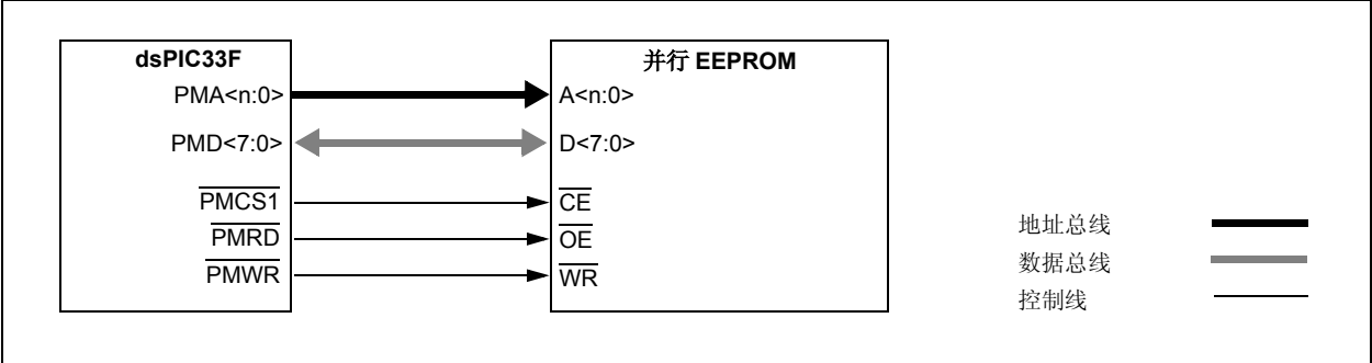
图 25-10: 并行 EEPROM 示例（最多 11 位地址，8 位数据）
