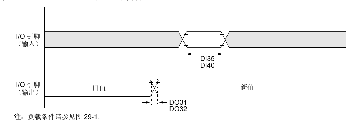
图 29-3: CLK0 和 I/O 时序特性
