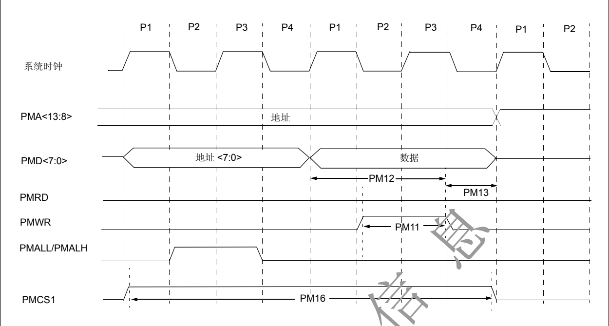
图 29-25: 并行主端口写时序图
