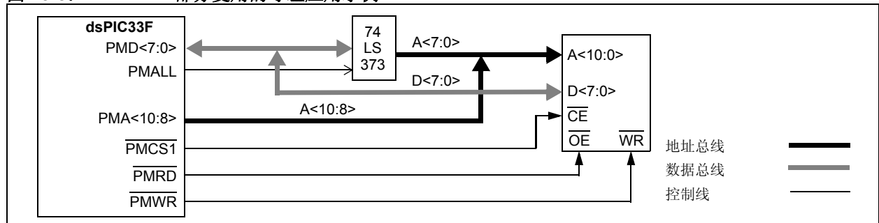
图 25-8: 部分复用的寻址应用示例
