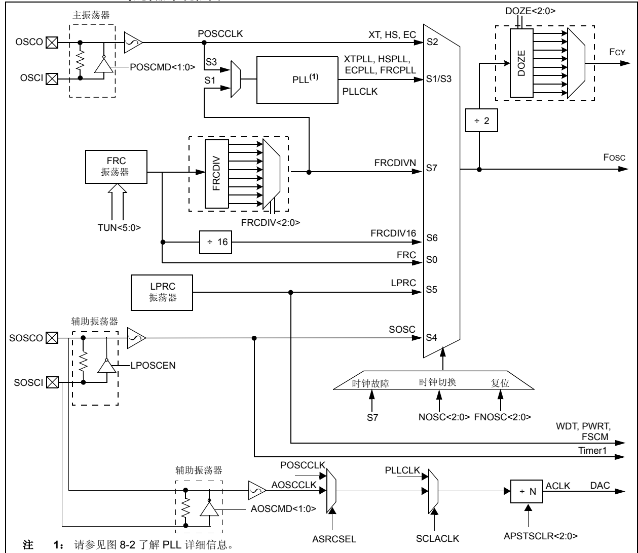
图 8-1: dsPIC33FJ32GP302/304、dsPIC33FJ64GPX02/X04 和 dsPIC33FJ128GPX02/X04 振荡器系统框图
