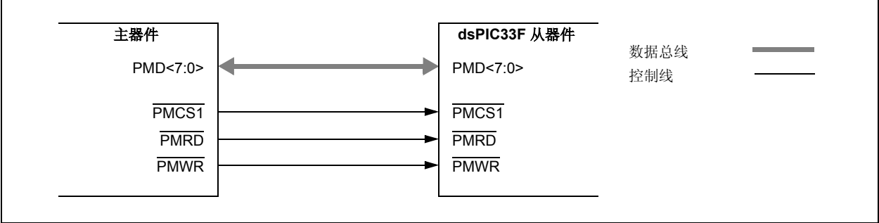
图 25-2: 传统并行从端口示例
