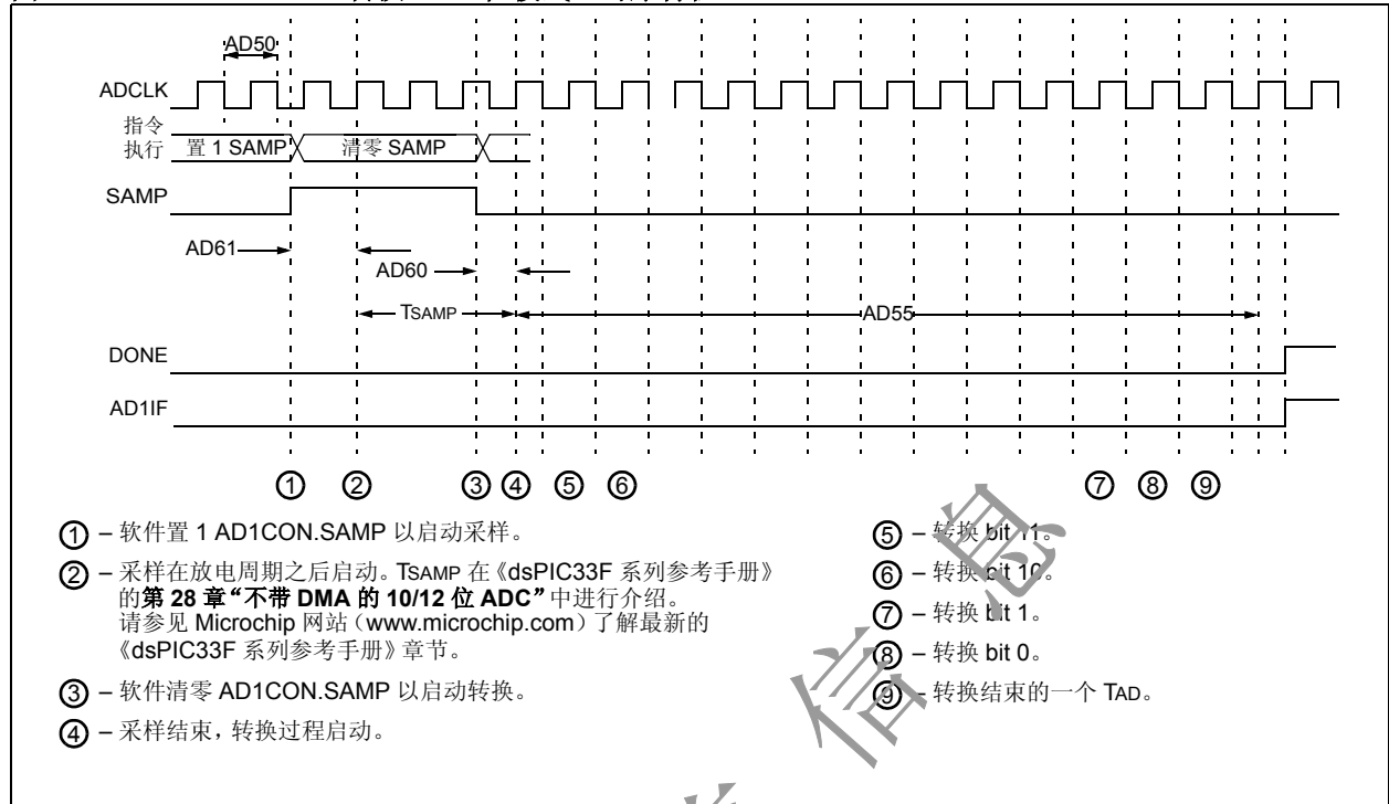
图 29-20: ADC 转换 (12 位模式) 时序特性 (ASAM = 0, SSRC&lt;2:0&gt; = 000)
