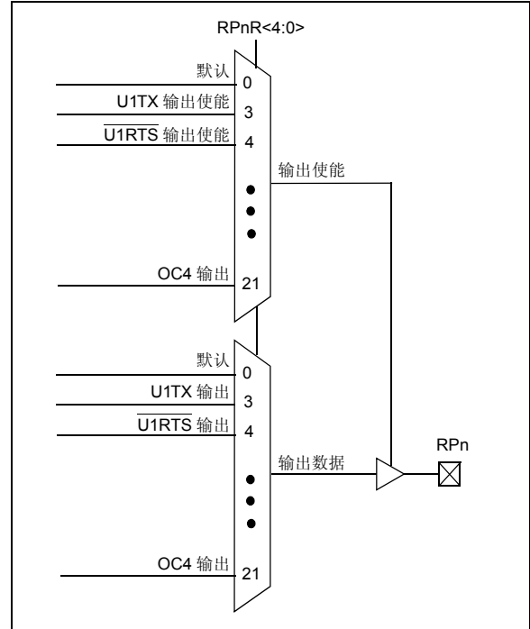
图 10-3: RPn 的可重映射输出的多路开关选择
