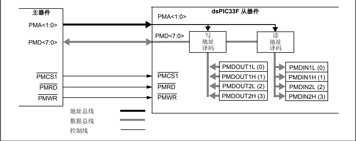
图 25-3: 可寻址的并行从端口示例
