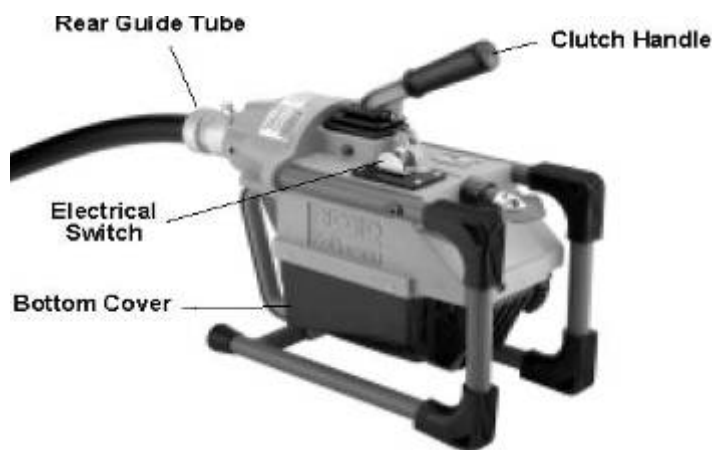
图 3 – K-60SP 疏通机
