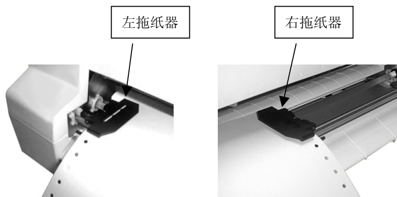
图 3-7 将连续纸安装在拖纸器上
