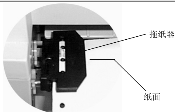
图 3-8 安装连续纸于拖纸器齿轮上
