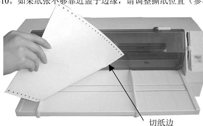
图 3-10 撕连续纸
