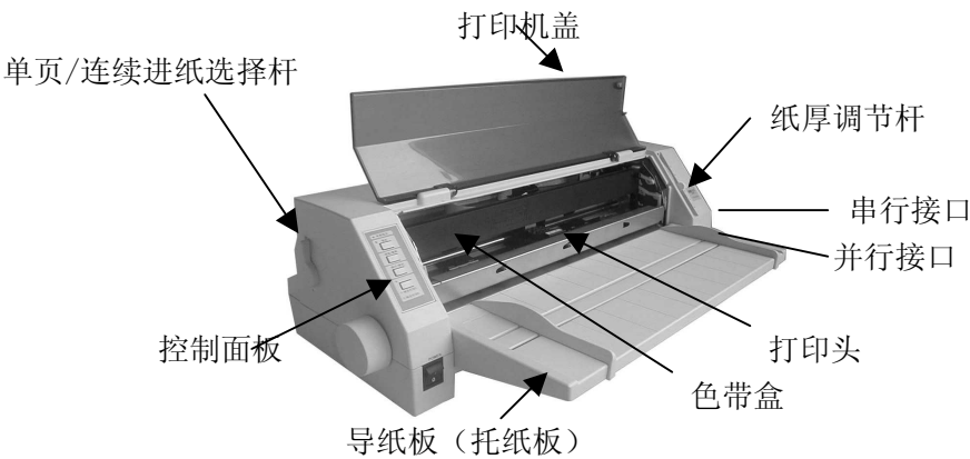
图 2-2 打印机主要部分（前视图）
