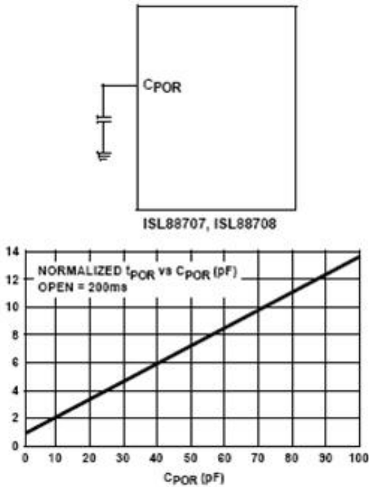
图3. 利用电容来调整 t_{POR}
