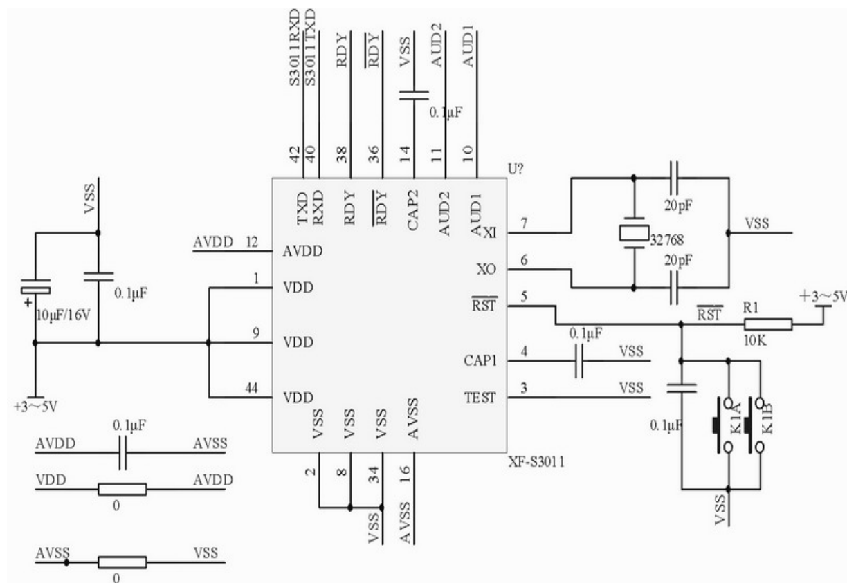
图表 5 XF-S3011 芯片外围电路
