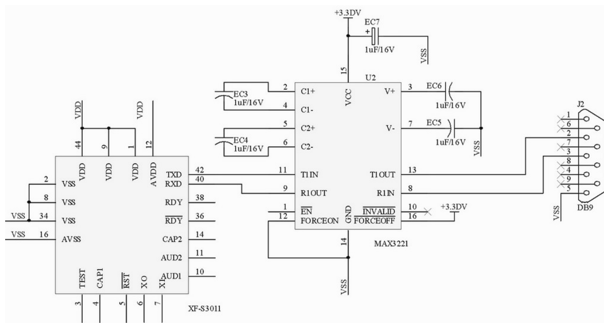
图表 7 XF-S3011 芯片以 PC 为上位机的连接
