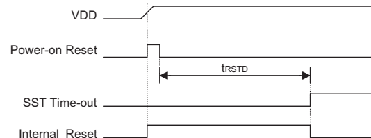
复位时序图
