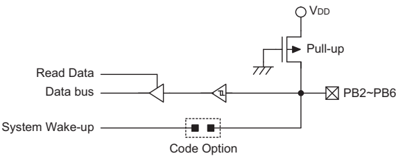
PB2~PB6 输入口
