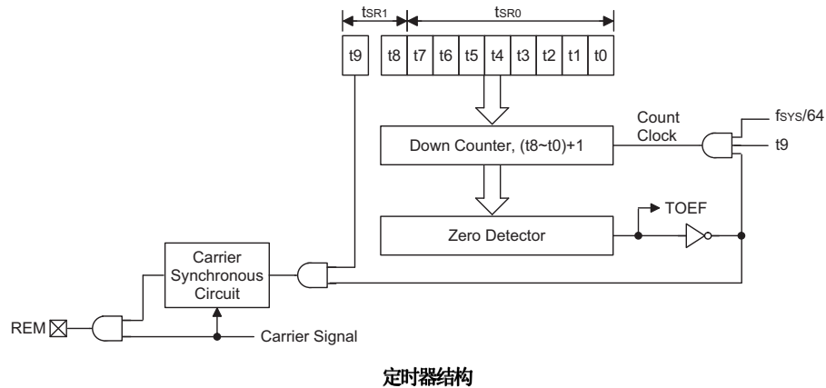
定时结构
