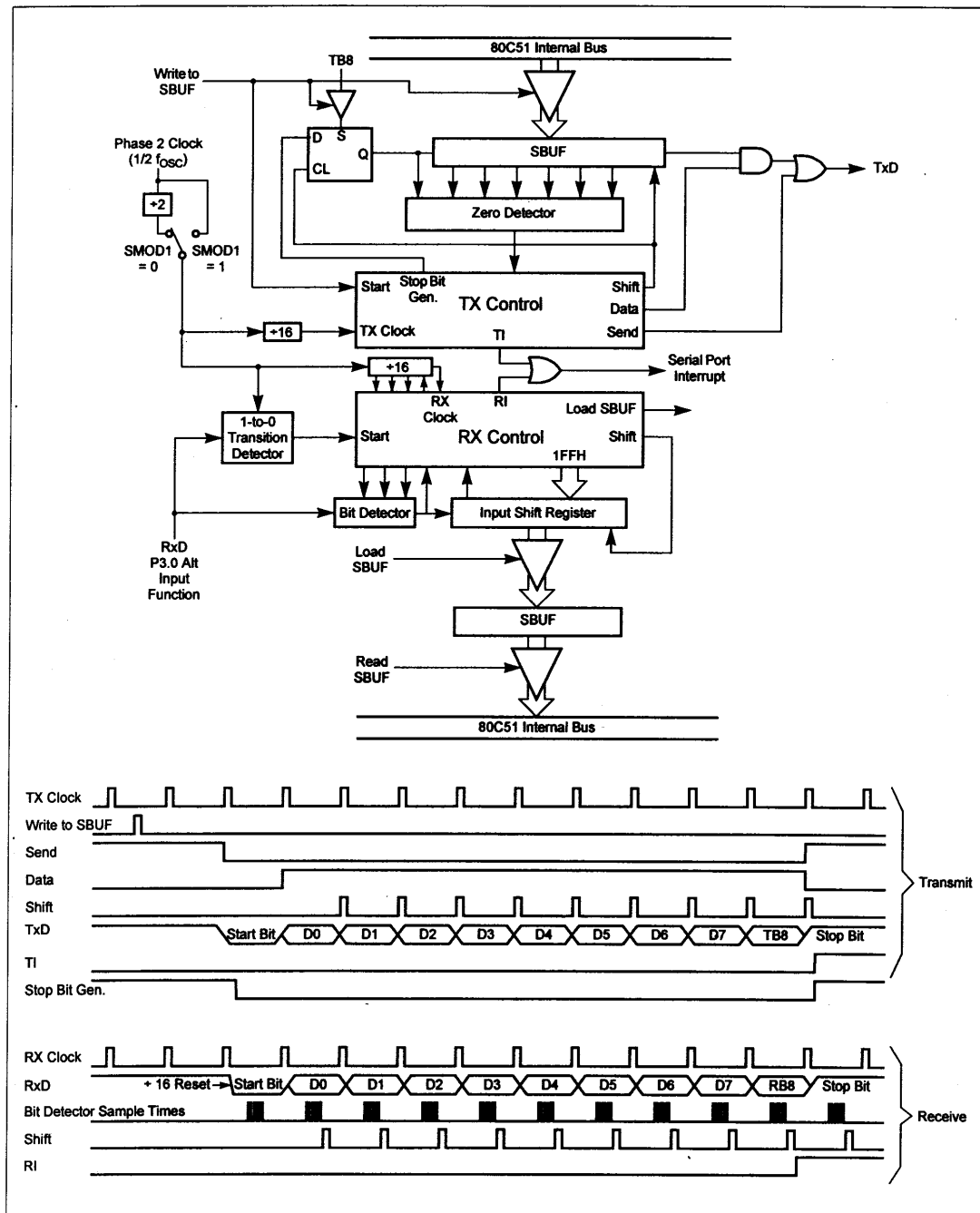
图 32 串口模式 2
