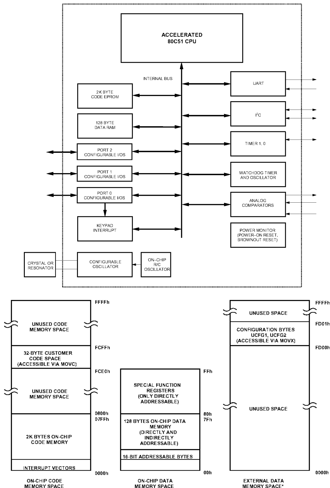
图1 P87LPC761 程序和数据存储器分布图
