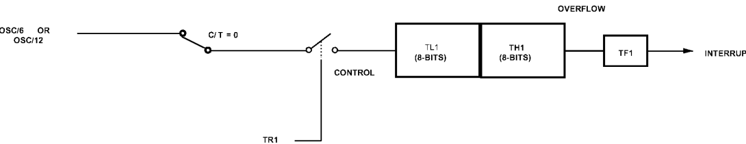
图 25 模式 1 时定时器 1 (16 位定时器)
