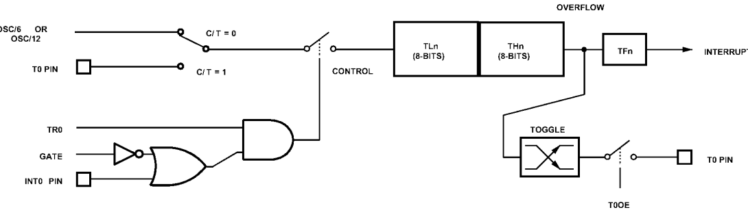
图 24 模式 1 时的定时/计数器 0 (16 位定时/计数器)
