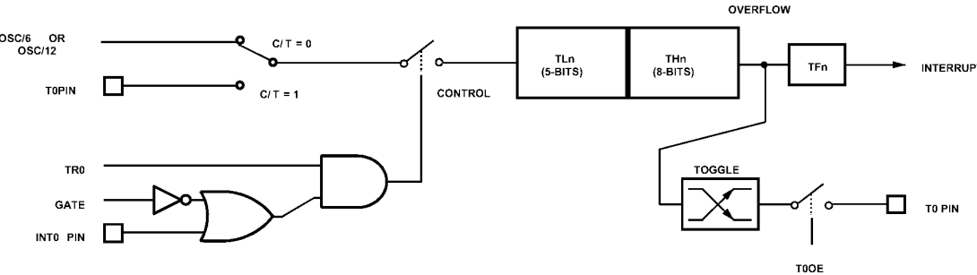
图 23 模式 0 时的定时/计数器 0 或 1 (13 位计数器)
