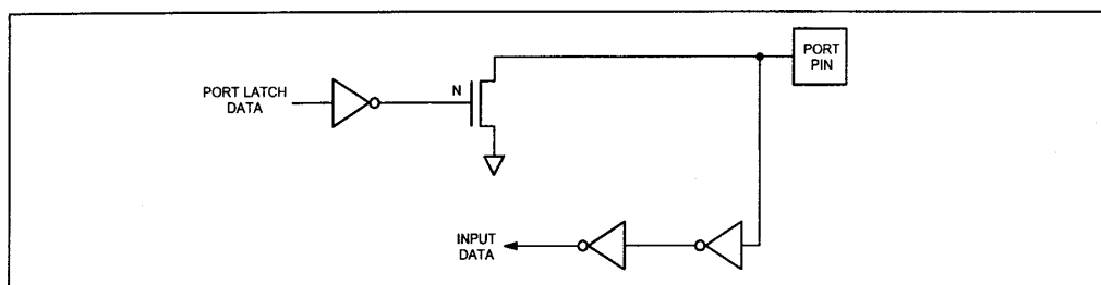
图 10 开漏输出
