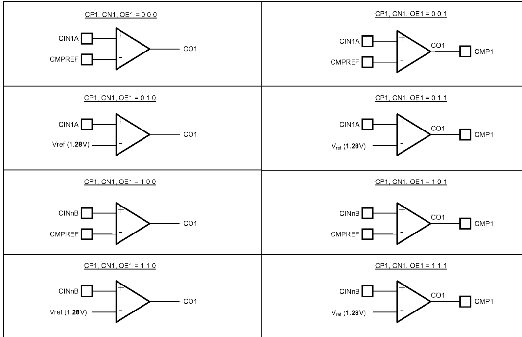
图 4 比较器配置
